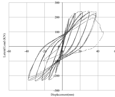
Kesme-Eğilme Göçmesi
