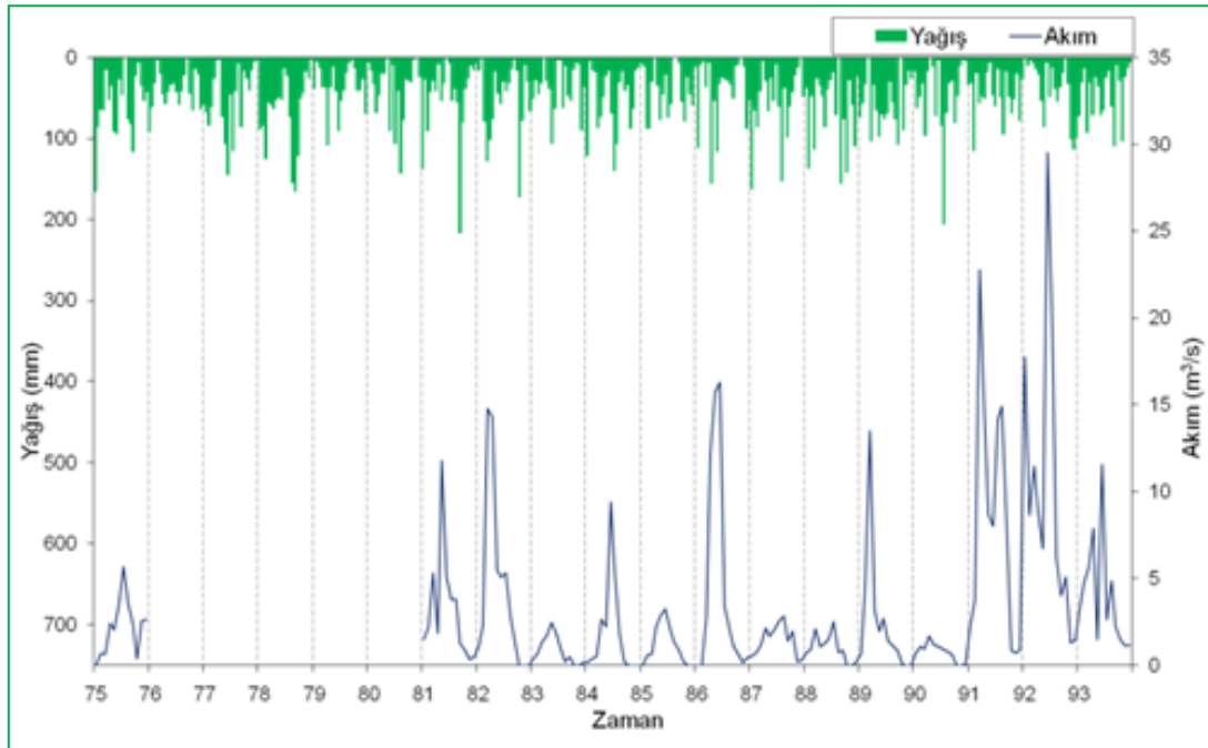
Şekil 2.3: Ergene Nehri Lüleburgaz Akım Gözlem İstasyonunda Gözlenen Akım ve Yağış Değerleri
