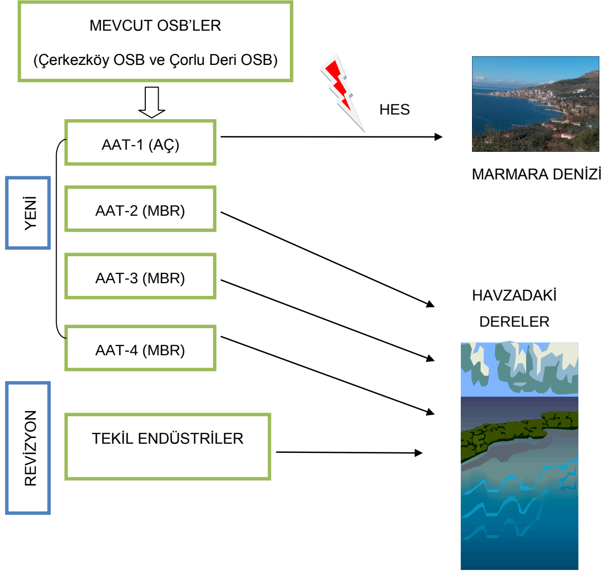
Şekil 7.11: 3. Alternatif Şematik Gösterimi
