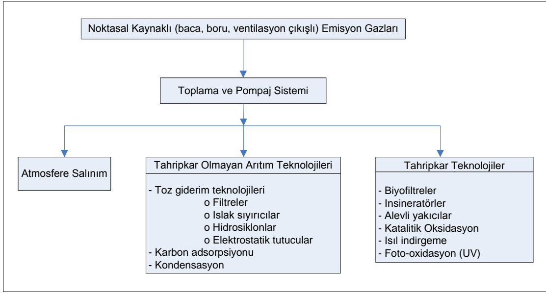
Şekil 2.4. Emisyon Gazları için Kullanılabilecek Genel Arıtım Seçenekleri
