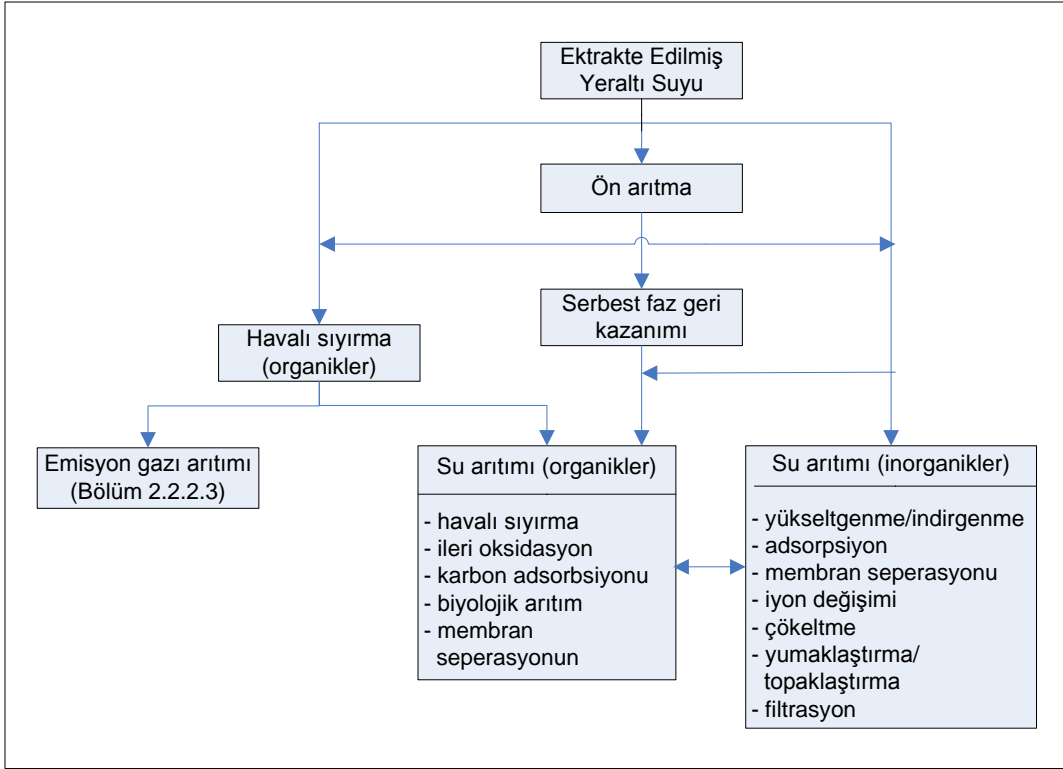
Şekil 2.3. Akiferden Ekstrakte Edilmiş Yeraltı Suyunun Arıtım Aşamaları ve Her Aşamada Kullanılabilecek Genel Arıtım Çeşitleri
