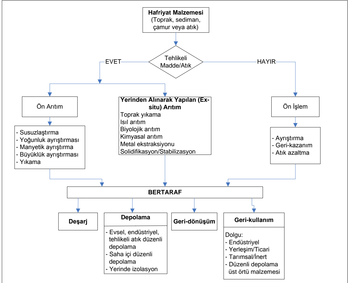
Şekil 2.2. Hafriyat Malzemesinin Yerinden Alınarak (Ex-Situ) Arıtımı/Temizlenmesi için Kullanılabilecek Seçenekler (Water Technology International Corp., 1997’den uyarlanmıştır).
