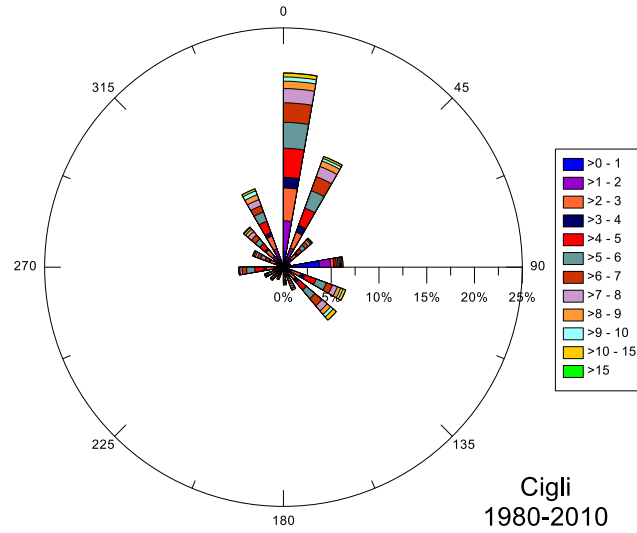
Şekil 12. Çiğli Meteoroloji İstasyonundan alınan saatlik rüzgar verileri (1980-2010) kullanılarak çizilen rüzgar gülü
