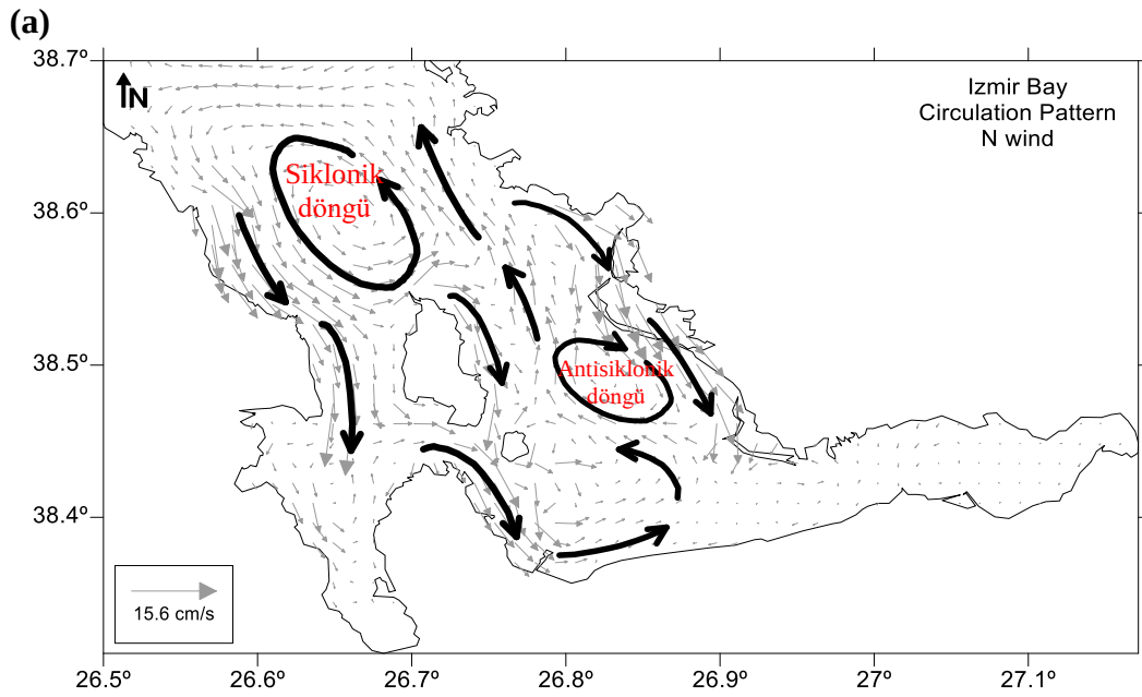
Şekil 13. İzmir Körfezi a) Genel akıntı deseni (Eronat, 2011) b) Şematik akıntı deseni (Oklar su kolonu boyunca net akıntıyı göstermektedir) (Eronat, 2017) .
