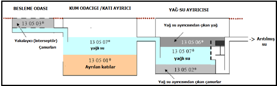
Şekil 5.1 :Kum odacıkları ve yağ separatörlerinden kaynaklanan atıklar
