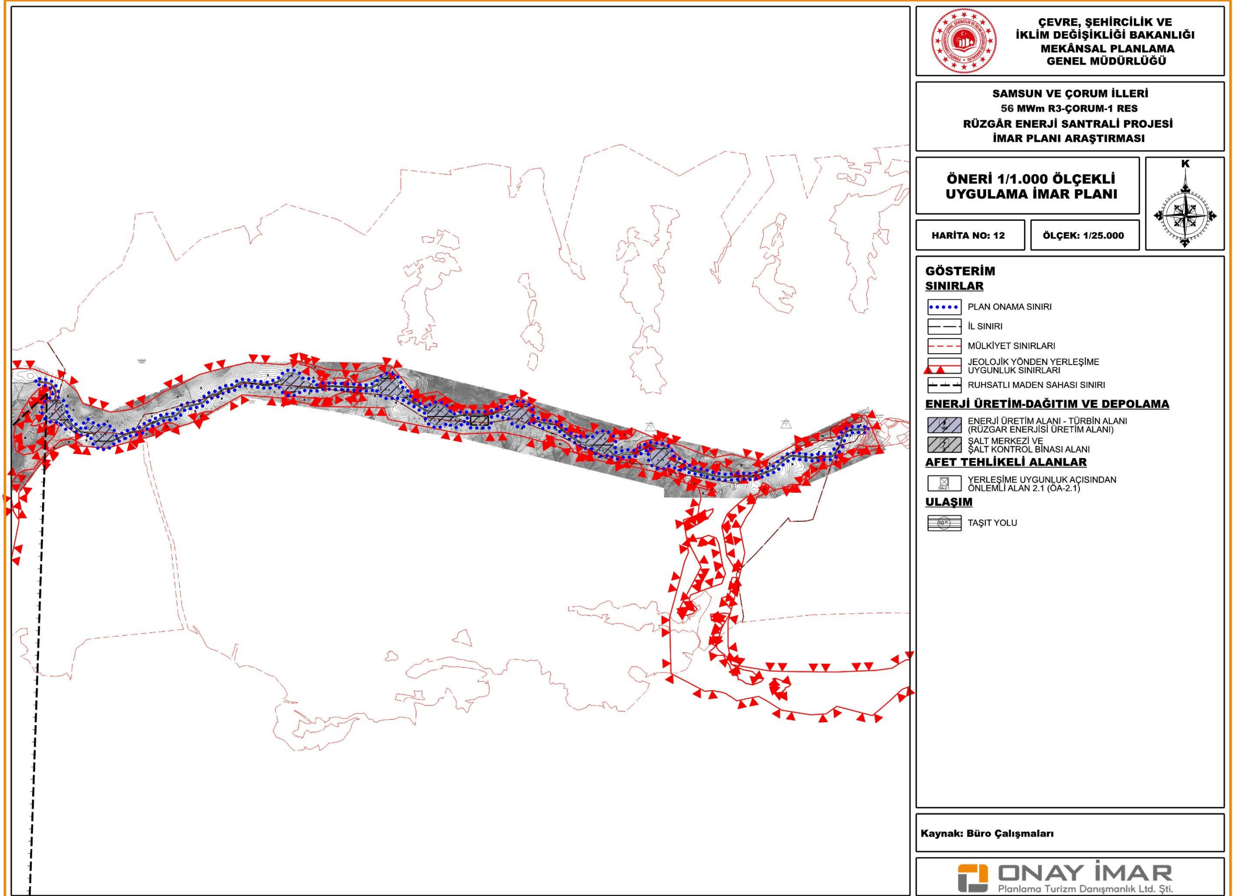
Harita 12: 56 MWM R3-Çorum-1 RES Rüzgâr Enerji Santrali Projesi 1/1.000 Ölçekli Uygulama İmar Planı
