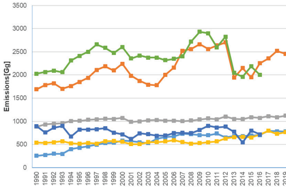
GRAFİK 112- KARAYOLU ULAŞIMINDAN KAYNAKLANAN NO x ve PM 10 EMİSYON TOPLAMLARI
