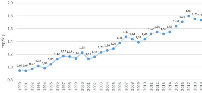
GRAFİK 126- YILLAR İTİBARIYLA KİŞİ BAŞINA ENERJİ TÜKETİMİ (tep/kişi)
