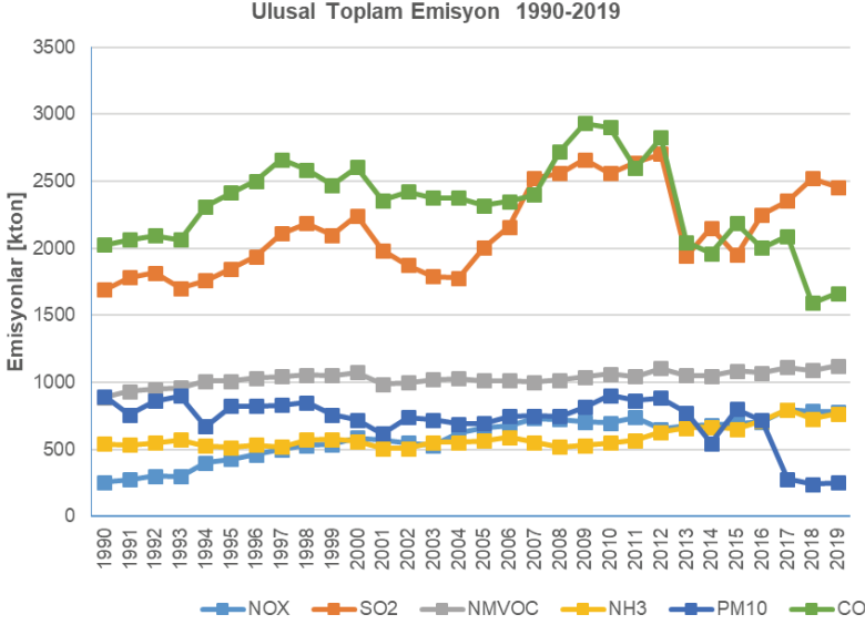
GRAFİK 24- SO 2 , NO x , NMVOC, NH 3 , CO ve PM 10 İÇİN EMİSYON TOPLAMLARI (1990-2019)
