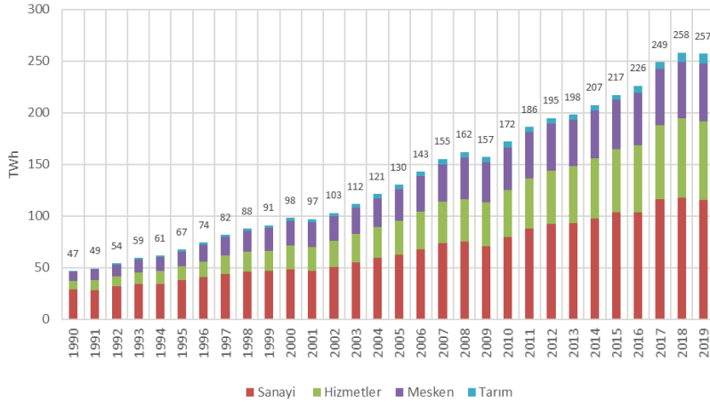
GRAFİK 125- YILLAR İTİBARIYLA SEKTÖRLERE GÖRE NET ELEKTRİK ENERJİSİ TÜKETİMİ (TWh)
