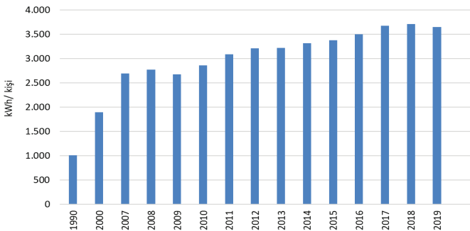
GRAFİK 127- KİŞİ BAŞI ELEKTRİK ENERJİSİ TÜKETİMİ (kWh/kişi)
