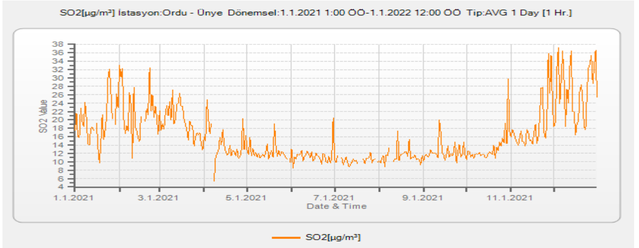
Grafik A.10 - Ünye İstasyonu SO 2 Parametresi Günlük Ortalama Değer Grafiği
