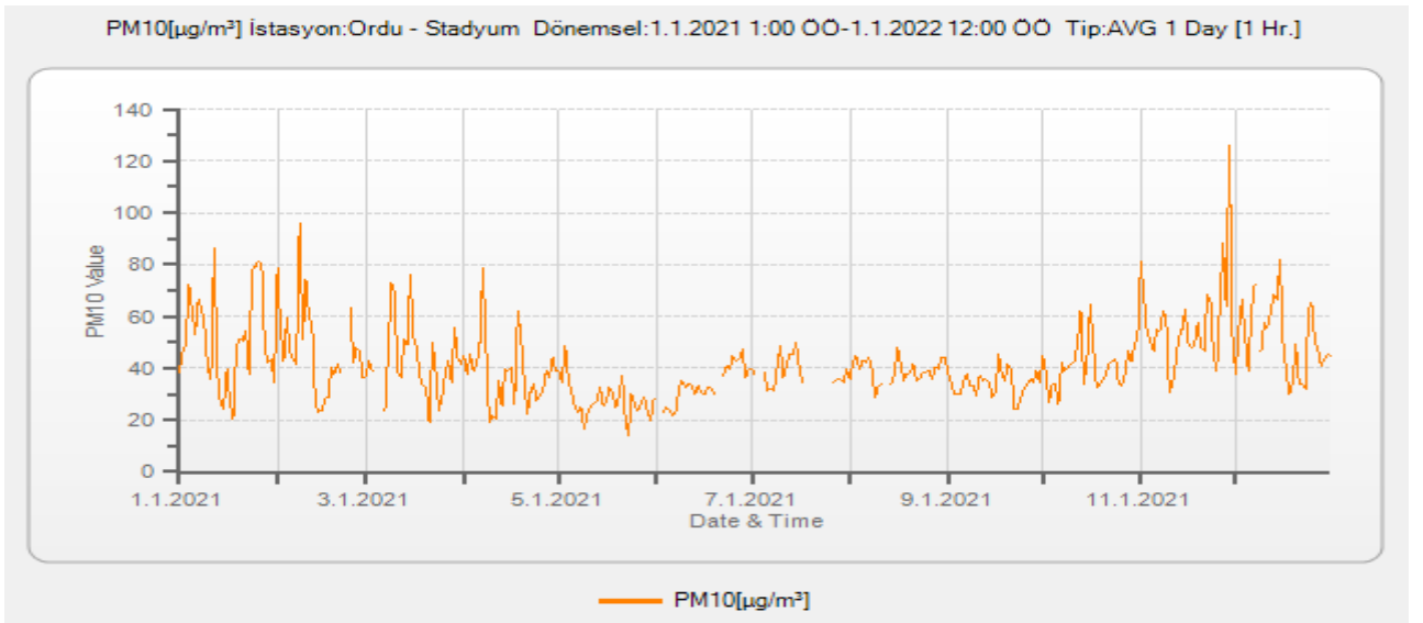
Grafik A.8- Stadyum İstasyonu PM 10 Parametresi Günlük Ortalama Değer Grafiği
