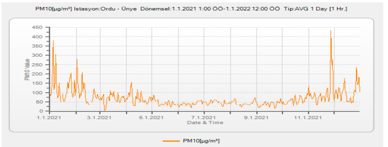
Grafik A.9- Ünye İstasyonu PM 10 Parametresi Günlük Ortalama Değer Grafiği
