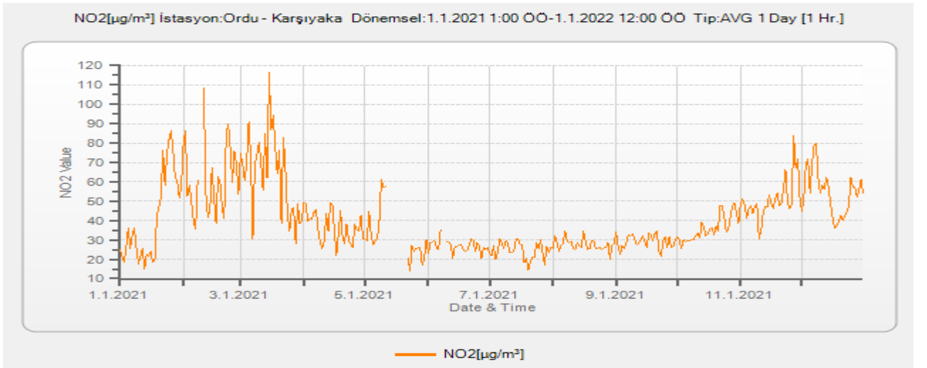
Grafik A.6- Karşıyaka İstasyonu NO 2 Parametresi Günlük Ortalama Değer Grafiği
