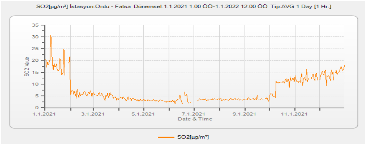
Grafik A.2- Fatsa İstasyonu SO 2 Parametresi Günlük Ortalama Değer Grafiği
