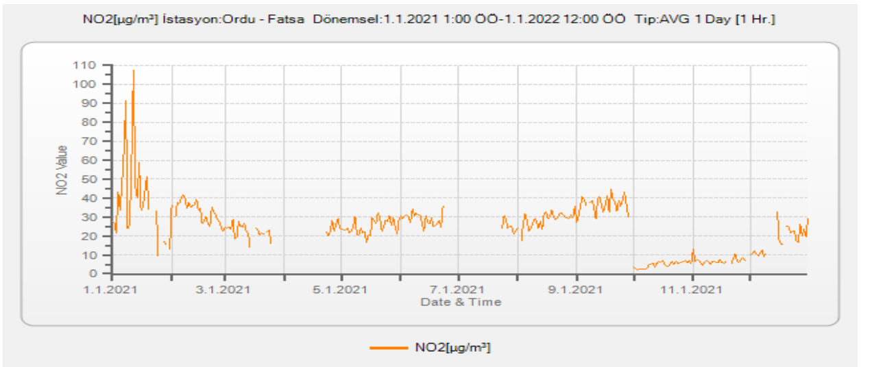
Grafik A.3- Fatsa İstasyonu NO 2 Parametresi Günlük Ortalama Değer Grafiği
