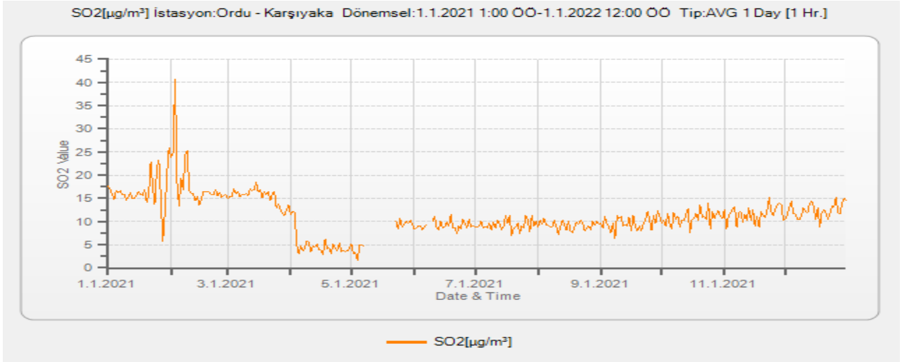
Grafik A.5- Karşıyaka İstasyonu SO 2 Parametresi Günlük Ortalama Değer Grafiği
