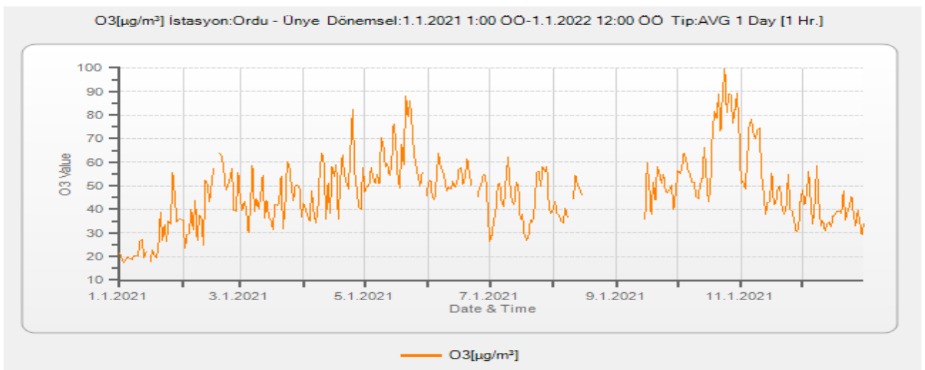
Grafik A.12- Ünye İstasyonu O 3 Parametresi Günlük Ortalama Değer Grafiği
