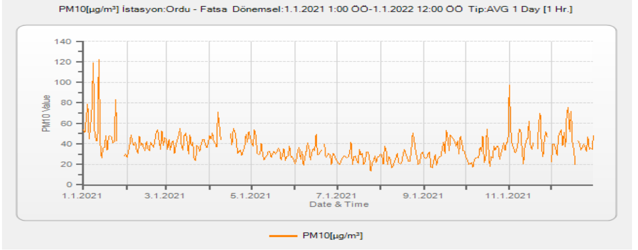
Grafik A.1- Fatsa İstasyonu PM 10 Parametresi Günlük Ortalama Değer Grafiği
