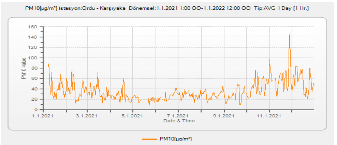
Grafik A.4- Karşıyaka İstasyonu PM 10 Parametresi Günlük Ortalama Değer Grafiği
