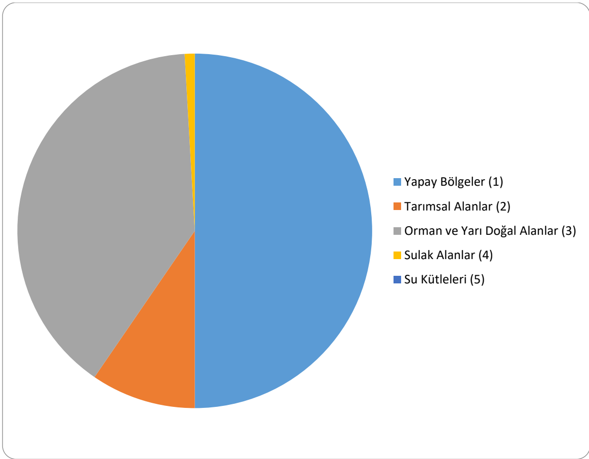
Grafik E.24 – Mardin ilinde 2022 yılı arazi kullanım durumuna göre arazi sınıflandırması
