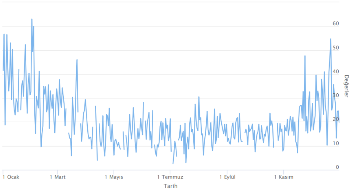
Grafik A.2 - 2022 yılında Mardin istasyonu SO 2 parametresi günlük ortalama değer grafiği* (havaizleme.gov.tr, 2023)
