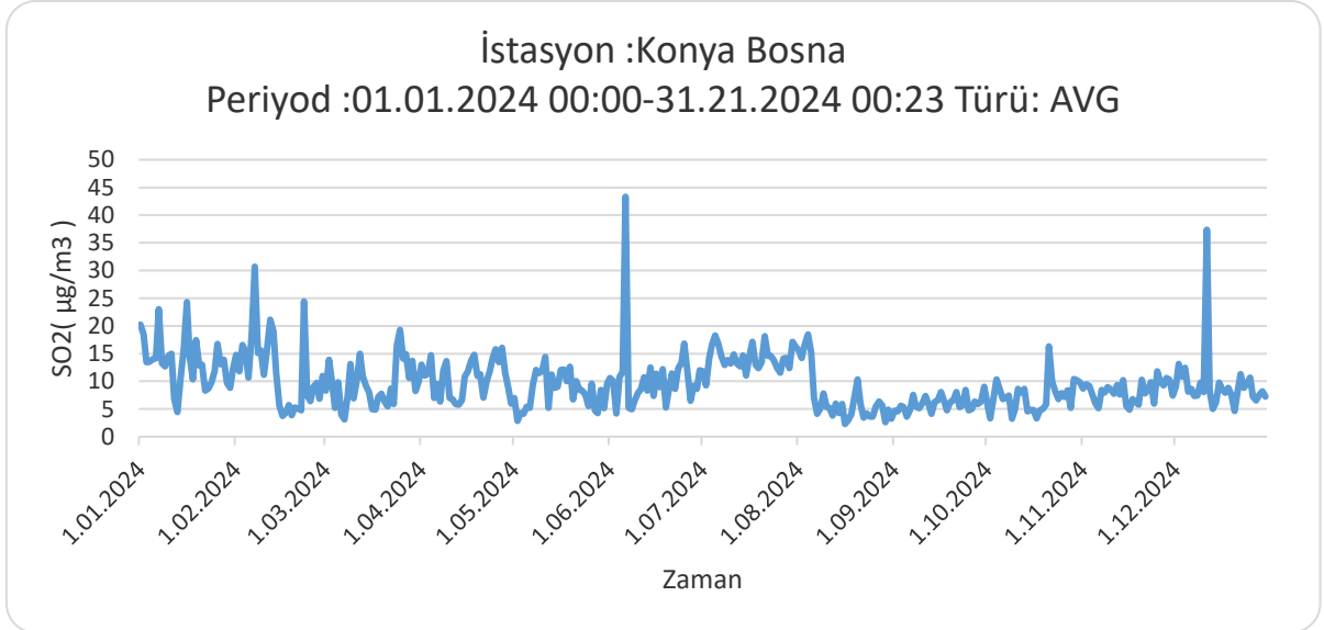
Grafik 10 - 2024 yılında Bosna istasyonu SO 2 parametresi günlük ortalama değer grafiği (Güney İç Anadolu Temiz Hava Merkezi Müdürlüğü, 2025)
