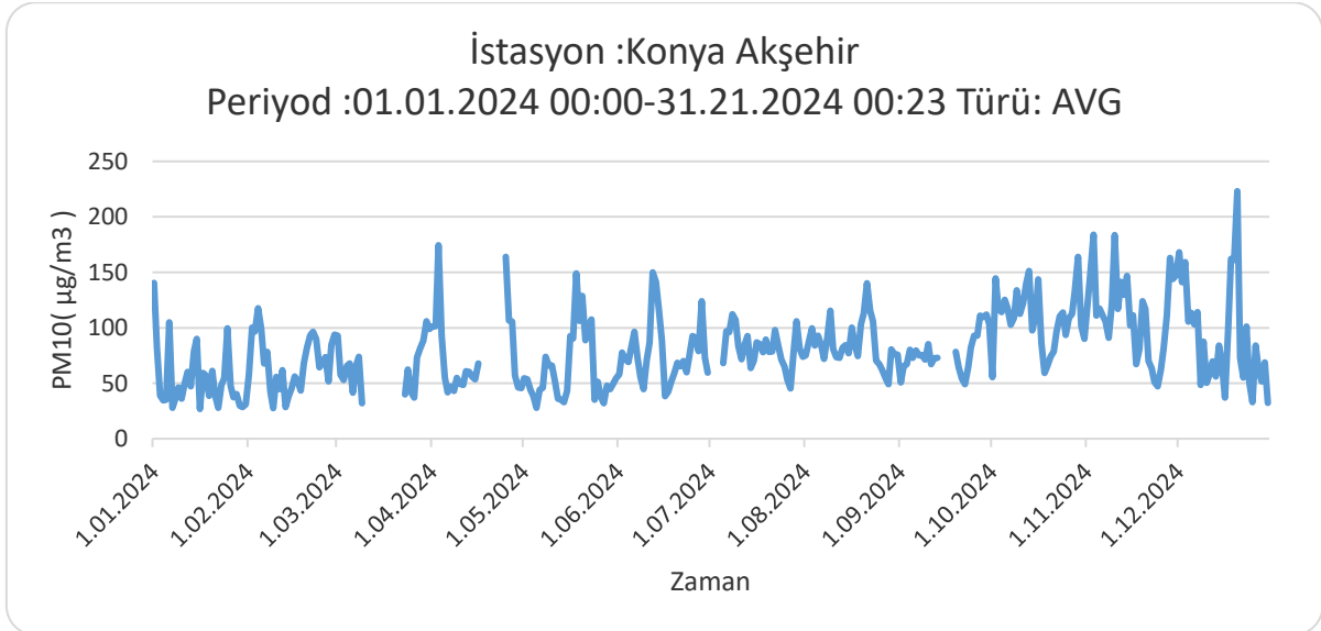
Grafik 1 - 2024 yılında Akşehir istasyonu PM 10 parametresi günlük ortalama değer grafiği (Güney İç Anadolu Temiz Hava Merkezi Müdürlüğü, 2025)
