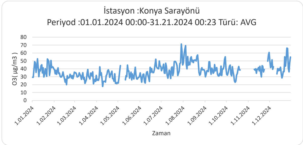
Grafik 17- 2024 yılında Sarayönü istasyonu O 3 parametresi günlük ortalama değeri grafiği* (Güney İç Anadolu Temiz Hava Merkezi Müdürlüğü, 2025)
