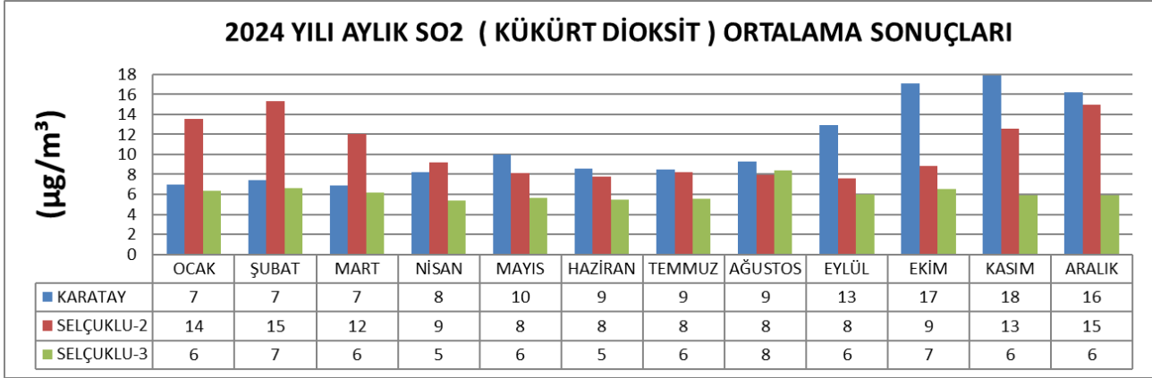
Grafik 18 - Konya ilinde 2024 yılında Karatay ve Selçuklu istasyonları SO 2 parametresi aylık ortalama değerler
