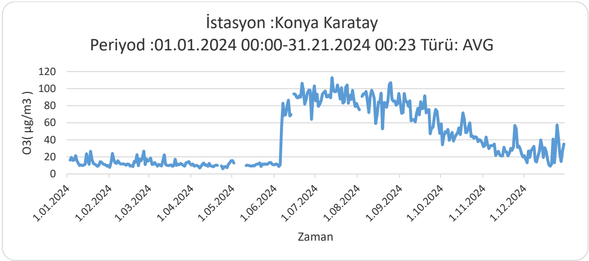
Grafik 12 - 2024 yılında Karatay istasyonu Ozon (O 3 ) parametresi günlük ortalama değer grafiği* (Güney İç Anadolu Temiz Hava Merkezi Müdürlüğü, 2025)
