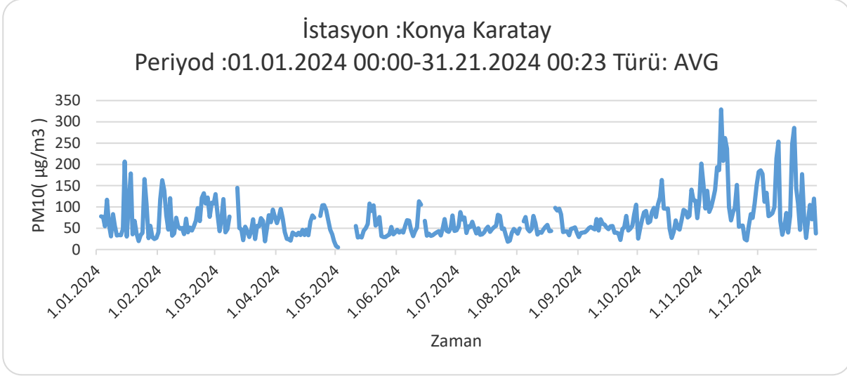
Grafik 2 – 2024 yılında Karatay istasyonu PM 10 parametresi günlük ortalama değeri grafiği (Güney İç Anadolu Temiz Hava Merkezi Müdürlüğü, 2025)
