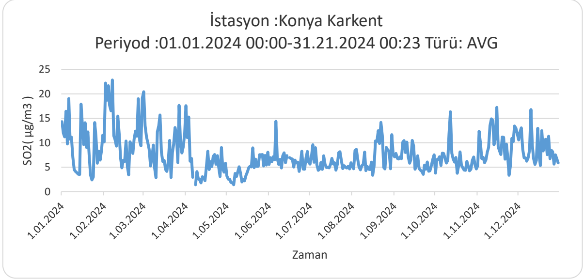
Grafik 9 - 2024 yılında Karkent istasyonu SO 2 parametresi günlük ortalama değer grafiği (Güney İç Anadolu Temiz Hava Merkezi Müdürlüğü, 2025)
