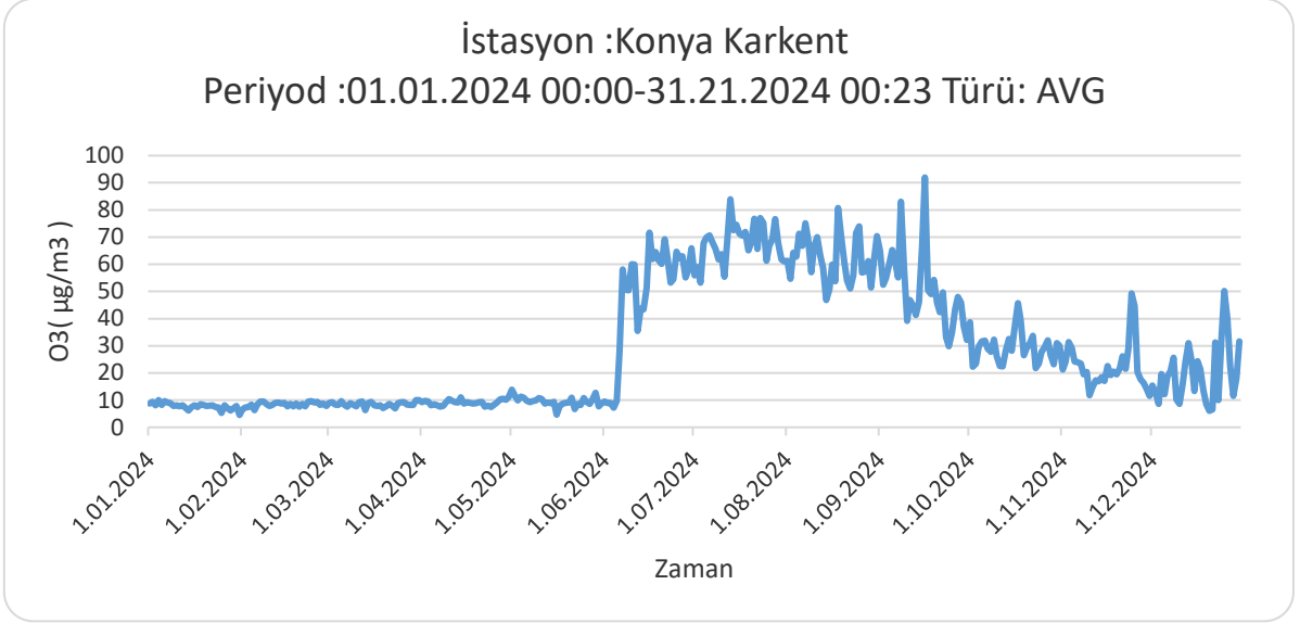
Grafik 14- 2024 yılında Karkent istasyonu O 3 parametresi günlük ortalama değer grafiği* (Güney İç Anadolu Temiz Hava Merkezi Müdürlüğü, 2025)
