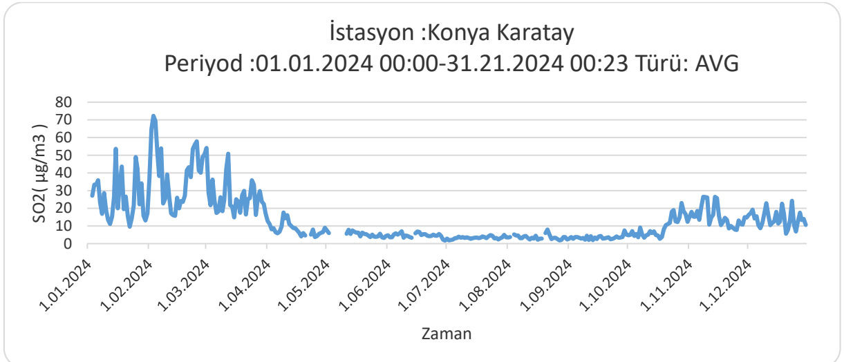
Grafik 8 - 2024 yılında Karatay istasyonu SO 2 parametresi günlük ortalama değer grafiği (Güney İç Anadolu Temiz Hava Merkezi Müdürlüğü, 2025)
