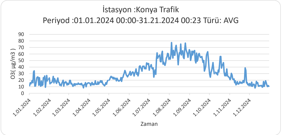
Grafik 15- 2024 yılında Trafik istasyonu O 3 parametresi günlük ortalama değer grafiği* (Güney İç Anadolu Temiz Hava Merkezi Müdürlüğü, 2025)
