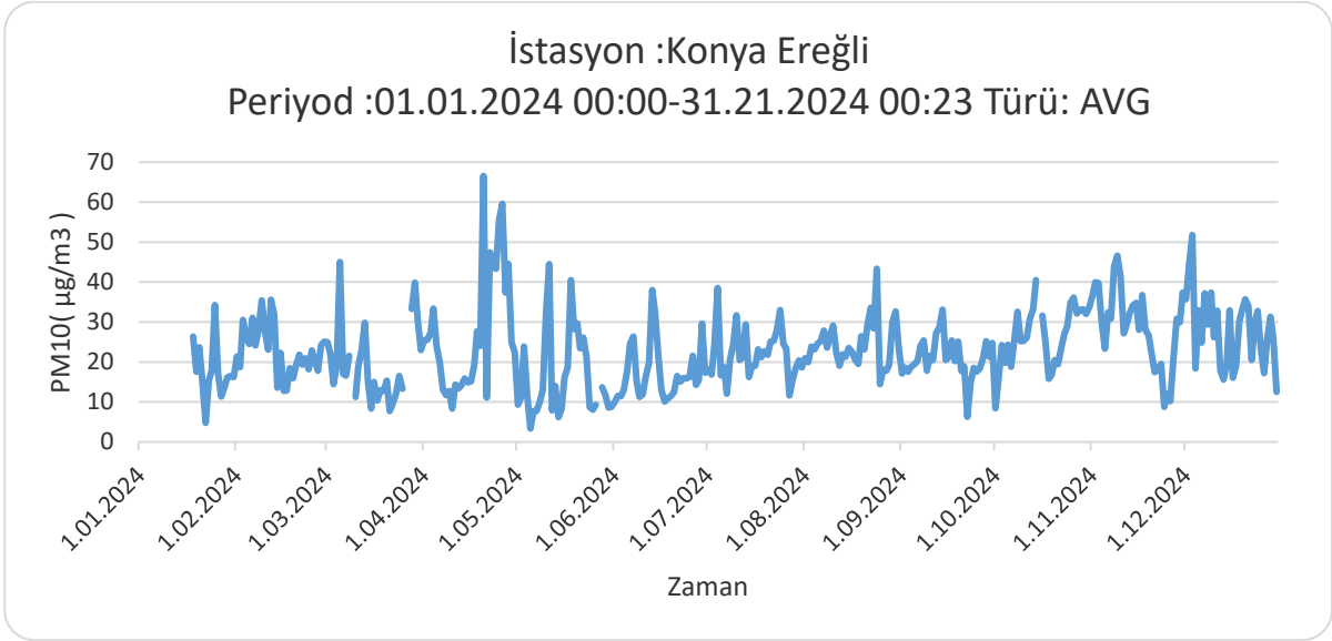
Grafik 4 yılında Ereğli istasyonu PM 10 parametresi günlük ortalama değer grafiği (Güney İç Anadolu Temiz Hava Merkezi Müdürlüğü, 2025)
