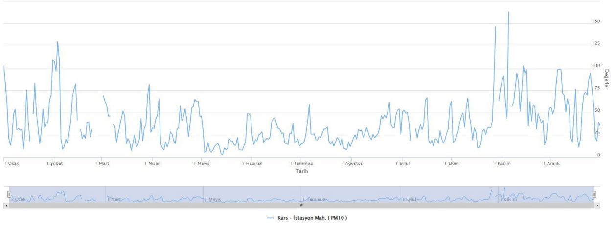
Grafik 1 - 2024 yılında Isınma istasyonu PM 10 parametresi günlük ortalama değer grafiği ( https://havaizleme.gov.tr , 2024)
