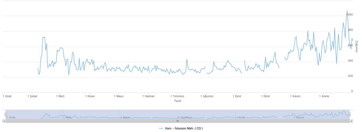
Grafik 7 - 2024 yılında Isınma istasyonu CO parametresi günlük ortalama değeri grafiği ( https://havaizleme.gov.tr , 2024)
