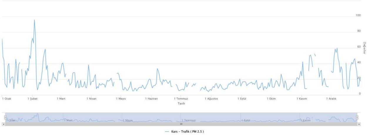
Grafik 9 - 2024 yılında Trafik istasyonu PM2,5 parametresi günlük ortalama değer grafiği ( https://havaizleme.gov.tr , 2024)
