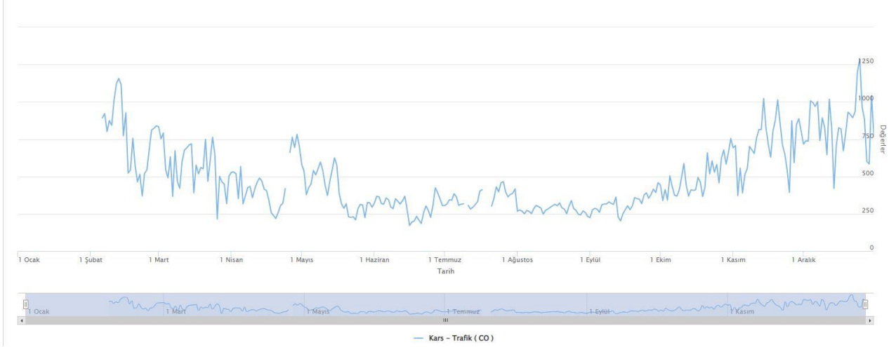
Grafik 13 - 2024 yılında Trafik istasyonu CO parametresi günlük ortalama değer grafiği ( https://havaizleme.gov.tr , 2024)
