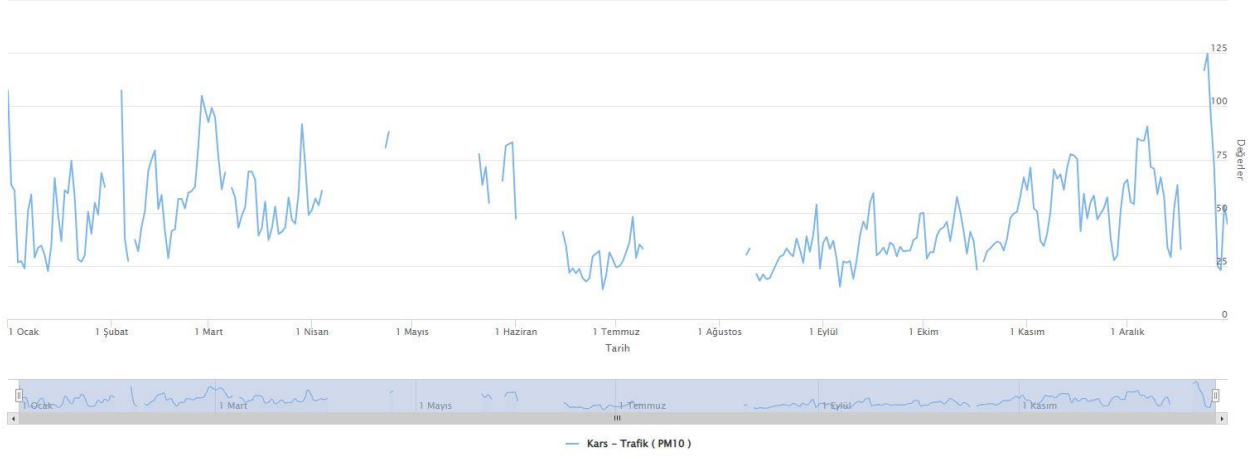
Grafik 10 - 2024 yılında Trafik istasyonu PM10 parametresi günlük ortalama değer grafiği ( https://havaizleme.gov.tr , 2024)
