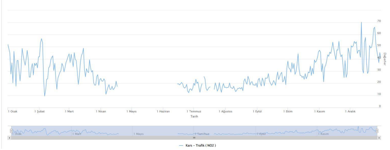
Grafik 12 - 2024 yılında Trafik istasyonu NO 2 parametresi günlük ortalama değer grafiği ( https://havaizleme.gov.tr , 2024)
