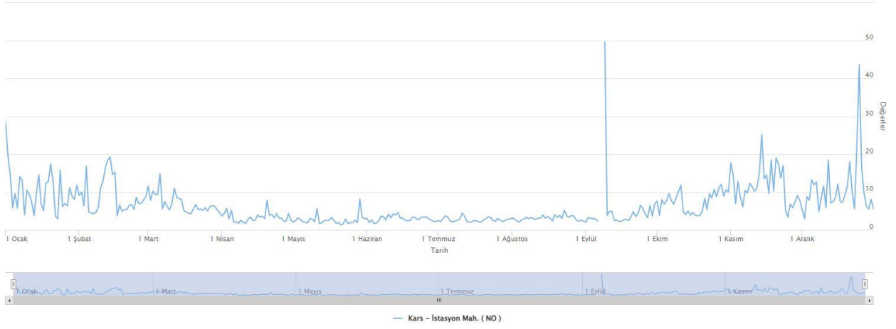
Grafik 3- 2024 yılında Isınma istasyonu NO parametresi günlük ortalama değer ( https://havaizleme.gov.tr , 2024)
