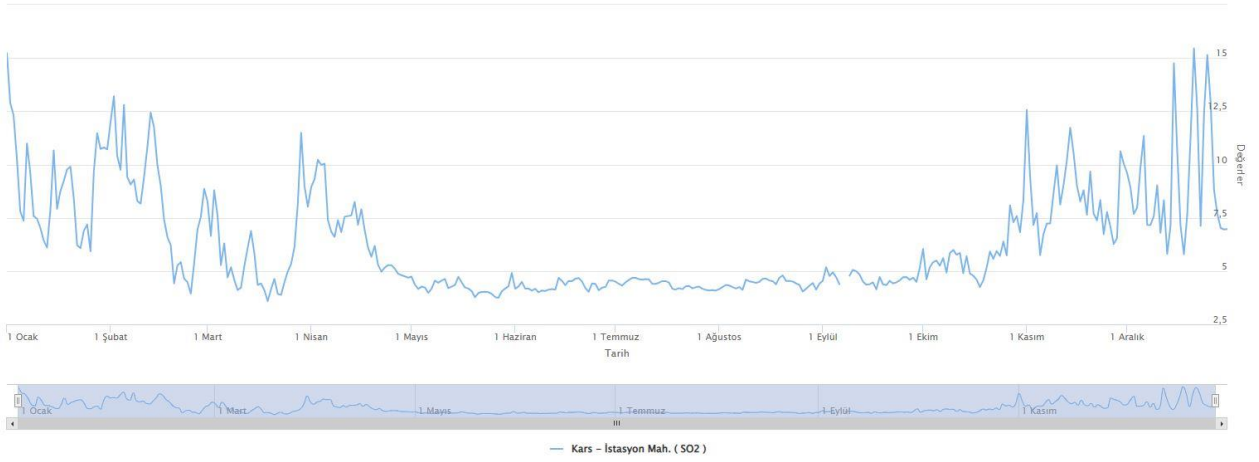
Grafik 2 - 2024 yılında Isınma istasyonu SO 2 parametresi günlük ortalama değer grafiği ( https://havaizleme.gov.tr , 2024)
