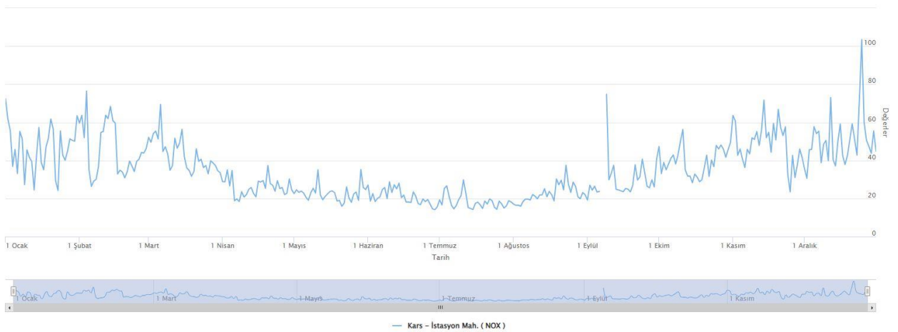
Grafik 5- 2024 yılında Isınma istasyonu NO x parametresi günlük ortalama değer grafiği ( https://havaizleme.gov.tr , 2024)
