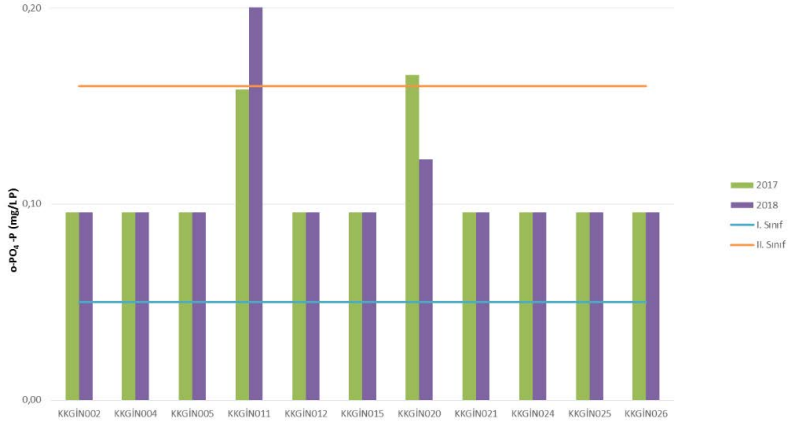
GRAFİK 45- KONYA KAPALI HAVZASI o-PO 4 -P (mg/L)
