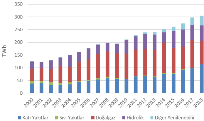
GRAFİK 107- KAYNAKLARA GÖRE TOPLAM ELEKTRİK ENERJİSİ ÜRETİMİ (TWh)
