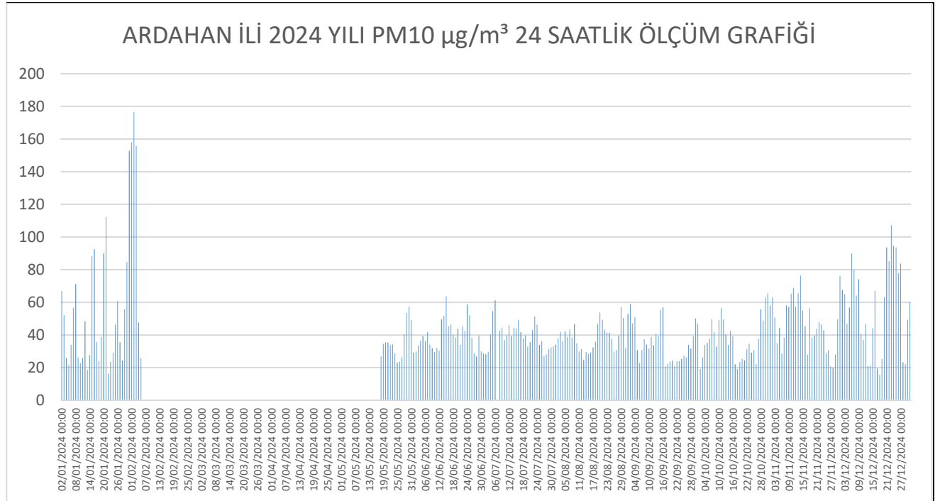
Grafik 1- 2024 yılında Ardahan istasyonu PM 10 parametresi günlük ortalama değer grafiği* (havaizleme.gov.tr, 2024)
