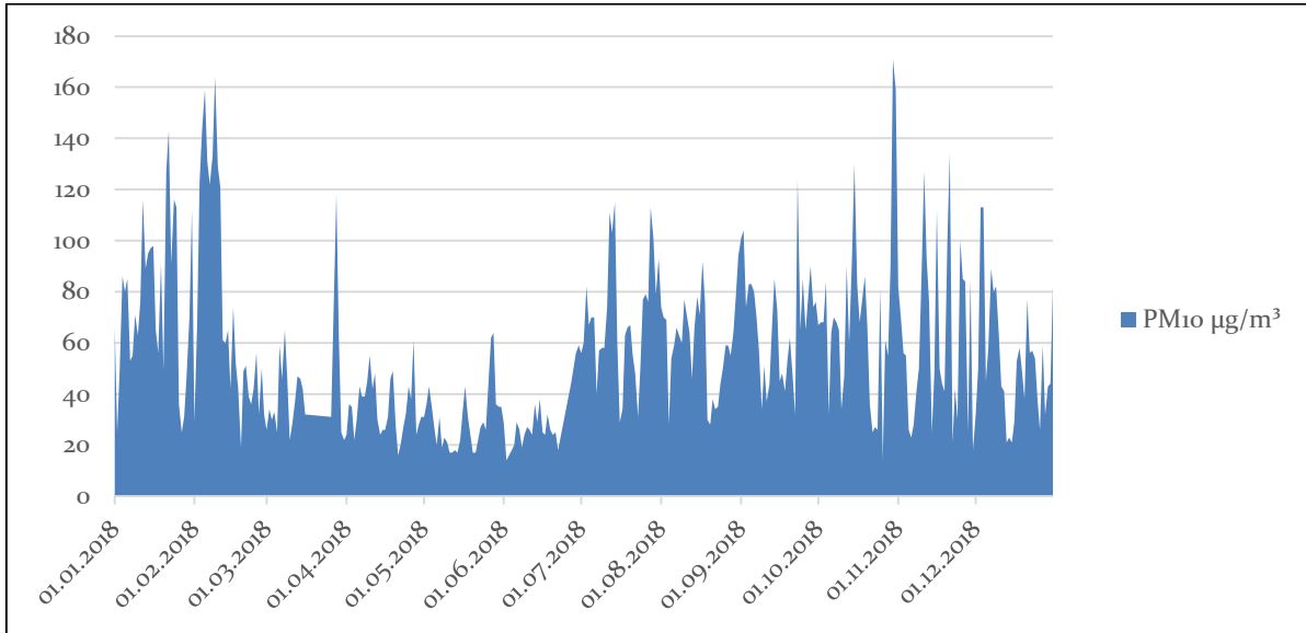
Grafik A.1 - Ağrı ili Merkez istasyonu PM 10 parametresi günlük ortalama değer grafiği
