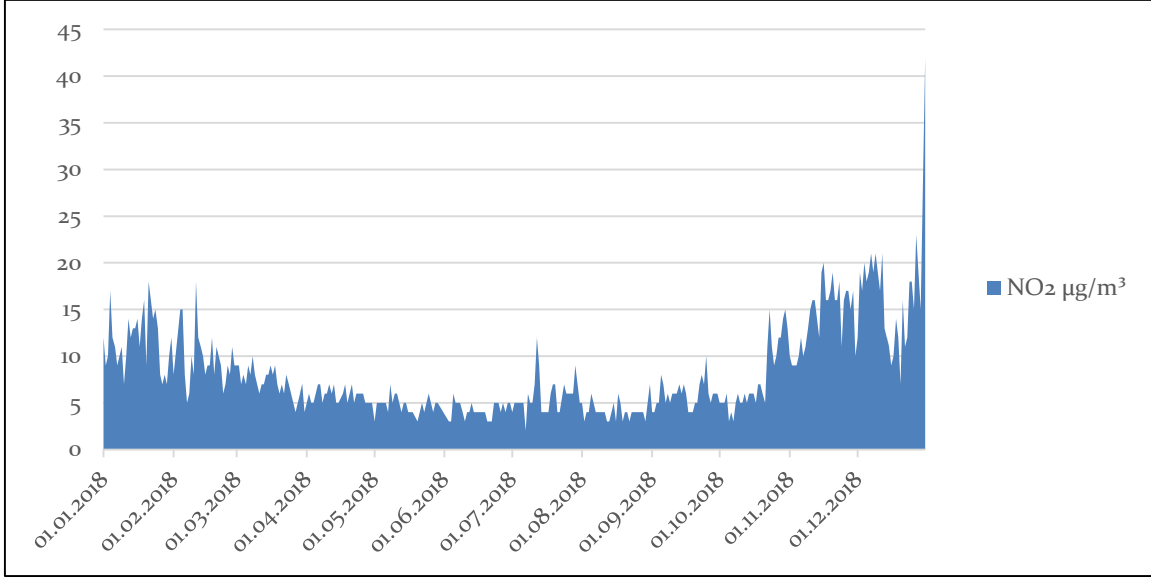
Grafik A.4 - Ağrı ili Merkez istasyonu NO 2 parametresi günlük ortalama değer grafiği (havaizleme.gov.tr, 2019)
