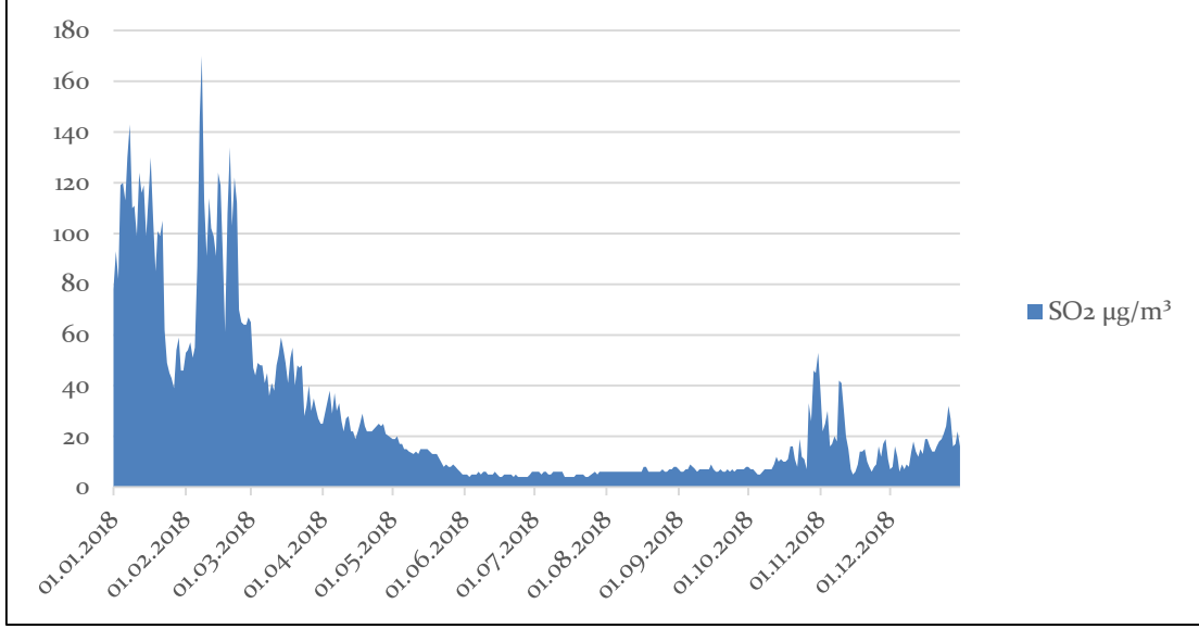
Grafik A.8 - Ağrı ili Doğubayazıt istasyonu SO 2 parametresi günlük ortalama değer grafiği (havaizleme.gov.tr, 2019)
