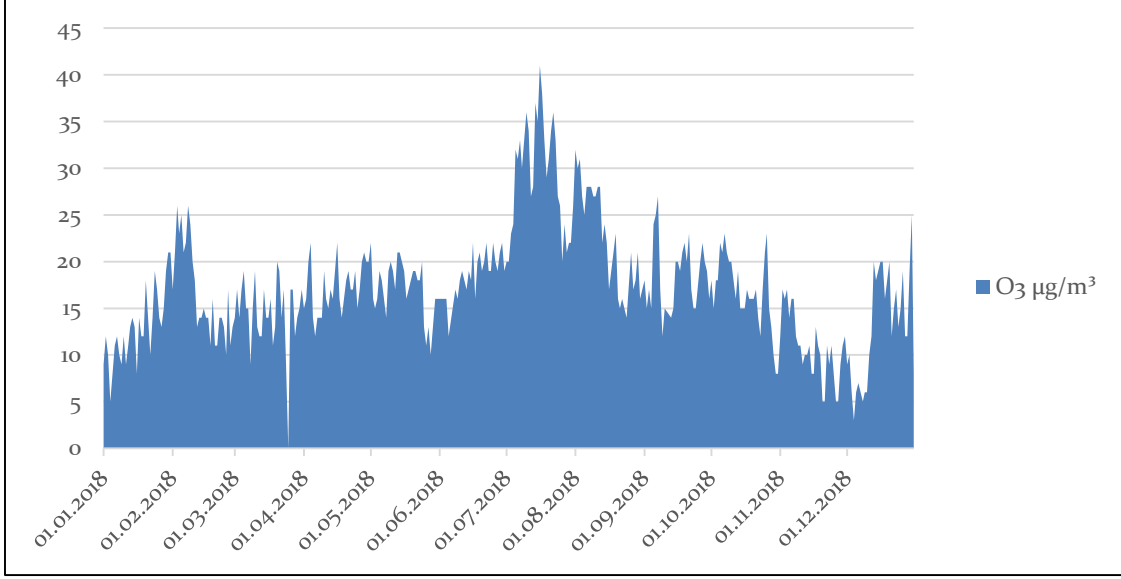
Grafik A.6 - Ağrı ili Merkez istasyonu O 3 parametresi günlük ortalama değer grafiği (havaizleme.gov.tr, 2019)
