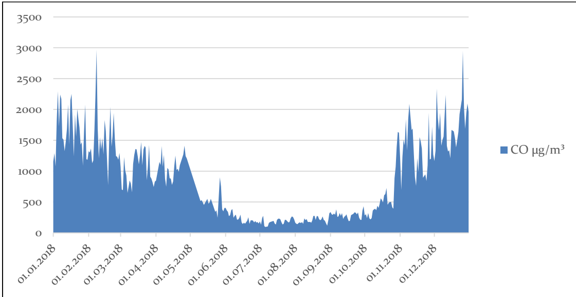
Grafik A.13 - Ağrı ili Doğubayazıt istasyonu CO parametresi günlük ortalama değer grafiği (havaizleme.gov.tr, 2019)
