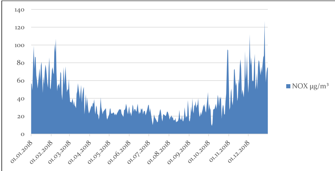
Grafik A.11 - Ağrı ili Doğubayazıt istasyonu NO x parametresi günlük ortalama değer grafiği (havaizleme.gov.tr, 2019)
