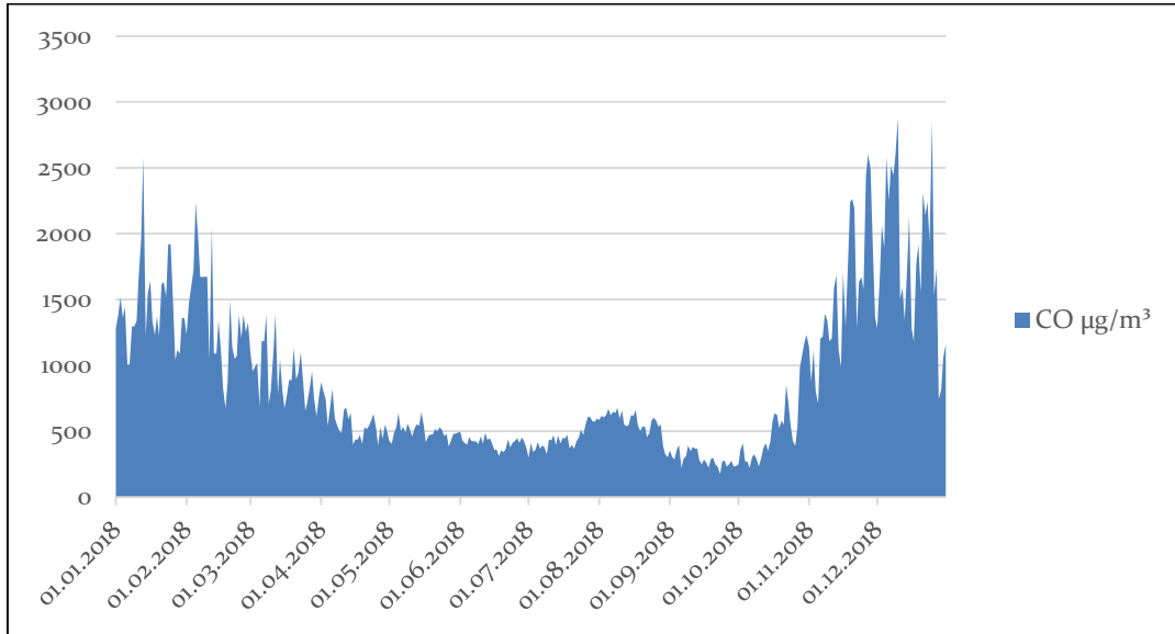
Grafik A.17 - Ağrı ili Patnos istasyonu CO parametresi günlük ortalama değer grafiği (havaizleme.gov.tr, 2019)
