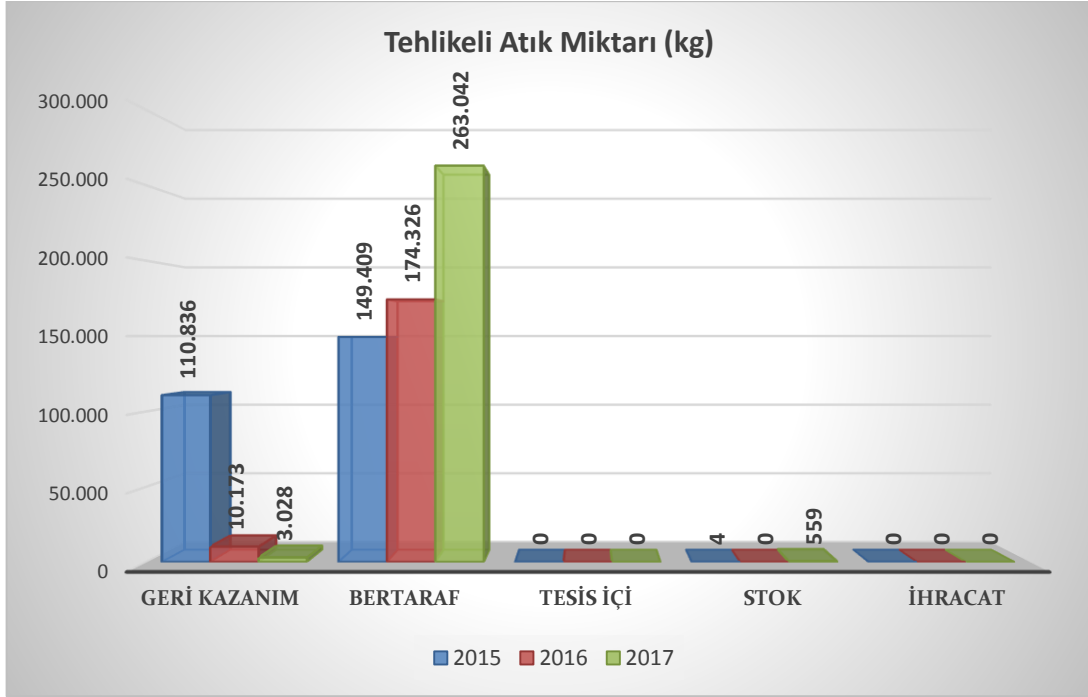
Grafik C.21 - Atık yönetim uygulaması verilerine göre ilimizdeki tehlikeli atık yönetimi (kg) (Atık Yönetim Uygulaması, 2019)
