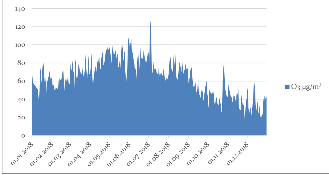
Grafik A.16 - Ağrı ili Patnos istasyonu O 3 parametresi günlük ortalama değer grafiği (havaizleme.gov.tr, 2019)
