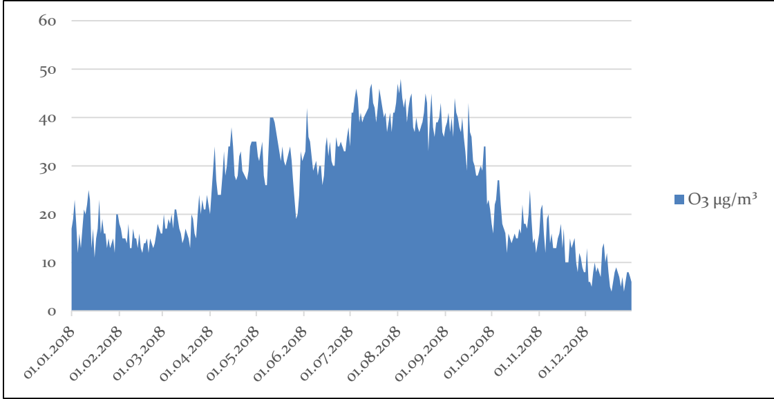
Grafik A.12 - Ağrı ili Doğubayazıt istasyonu O 3 parametresi günlük ortalama değer grafiği (havaizleme.gov.tr, 2019)
