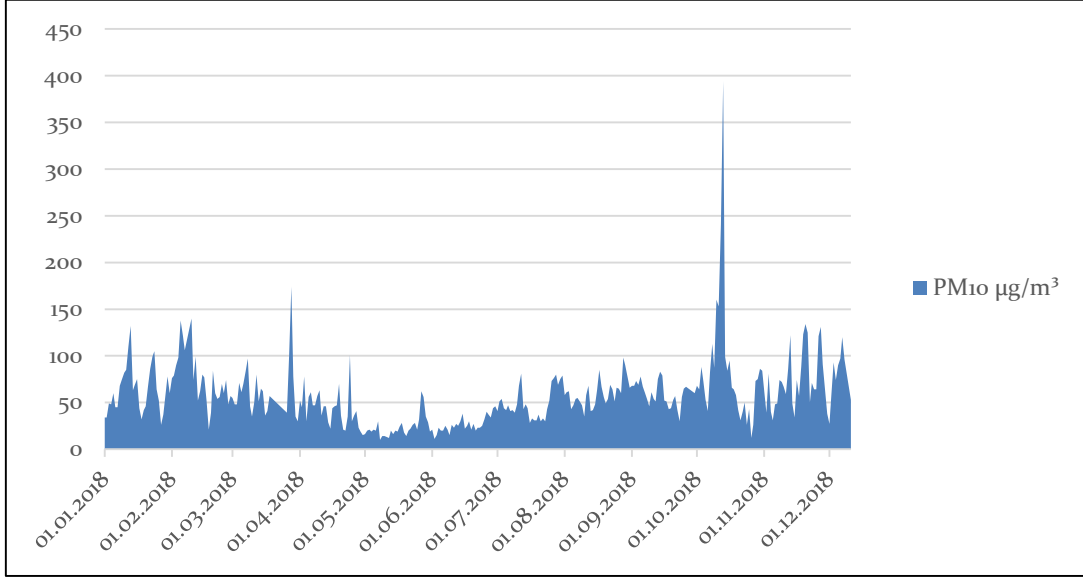
Grafik A.14 - Ağrı ili Patnos istasyonu PM 10 parametresi günlük ortalama değer grafiği (havaizleme.gov.tr, 2019)
