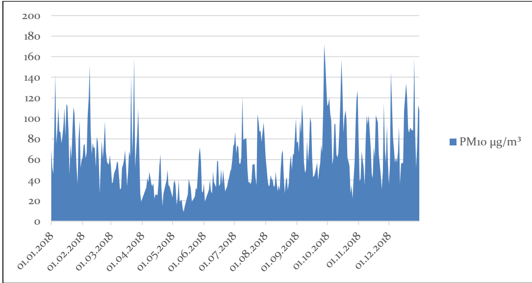
Grafik A.7 - Ağrı ili Doğubayazıt istasyonu PM 10 parametresi günlük ortalama değer grafiği (havaizleme.gov.tr, 2019)
