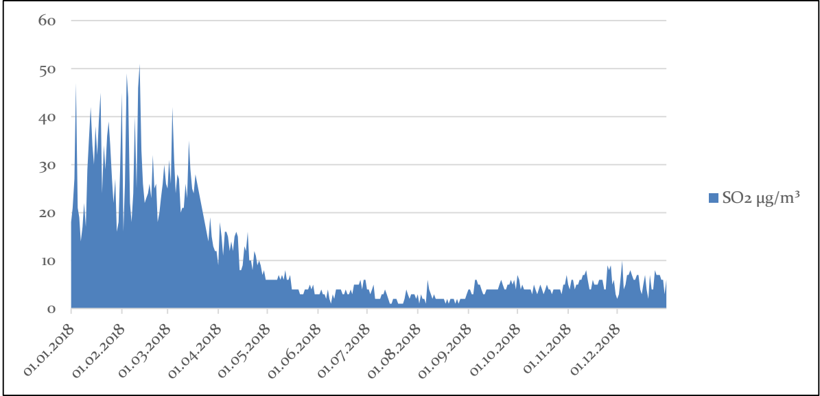
Grafik A.2 - Ağrı ili Merkez istasyonu SO 2 parametresi günlük ortalama değer grafiği (havaizleme.gov.tr, 2019)
