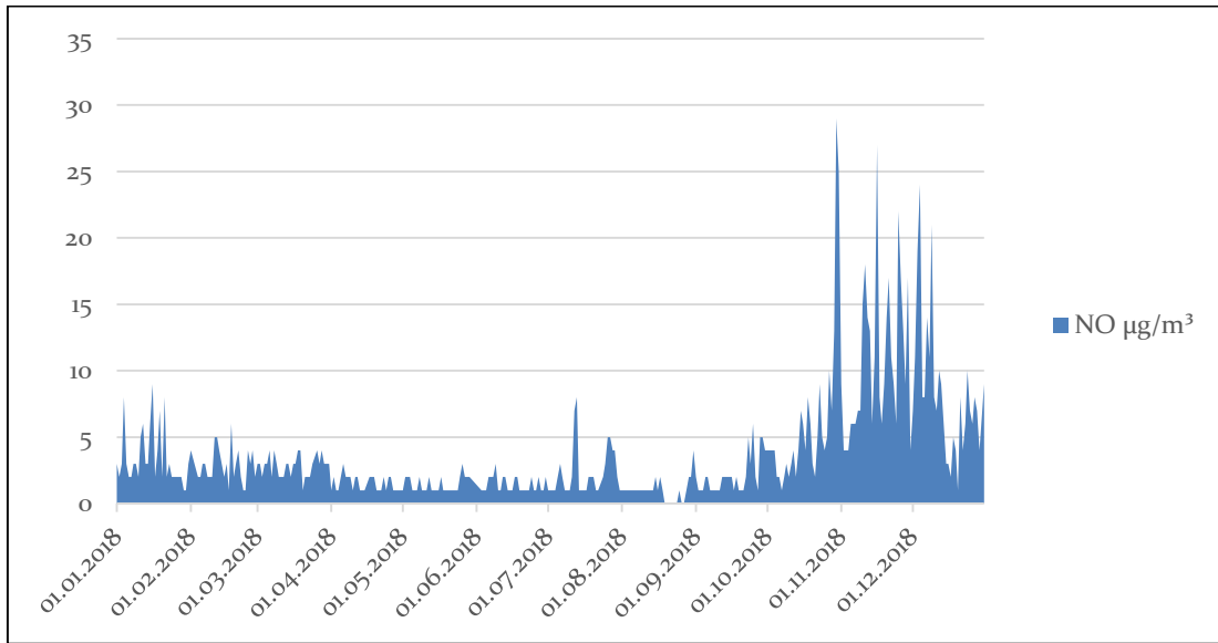
Grafik A.3 - Ağrı ili Merkez istasyonu NO parametresi günlük ortalama değer grafiği (havaizleme.gov.tr, 2019)
