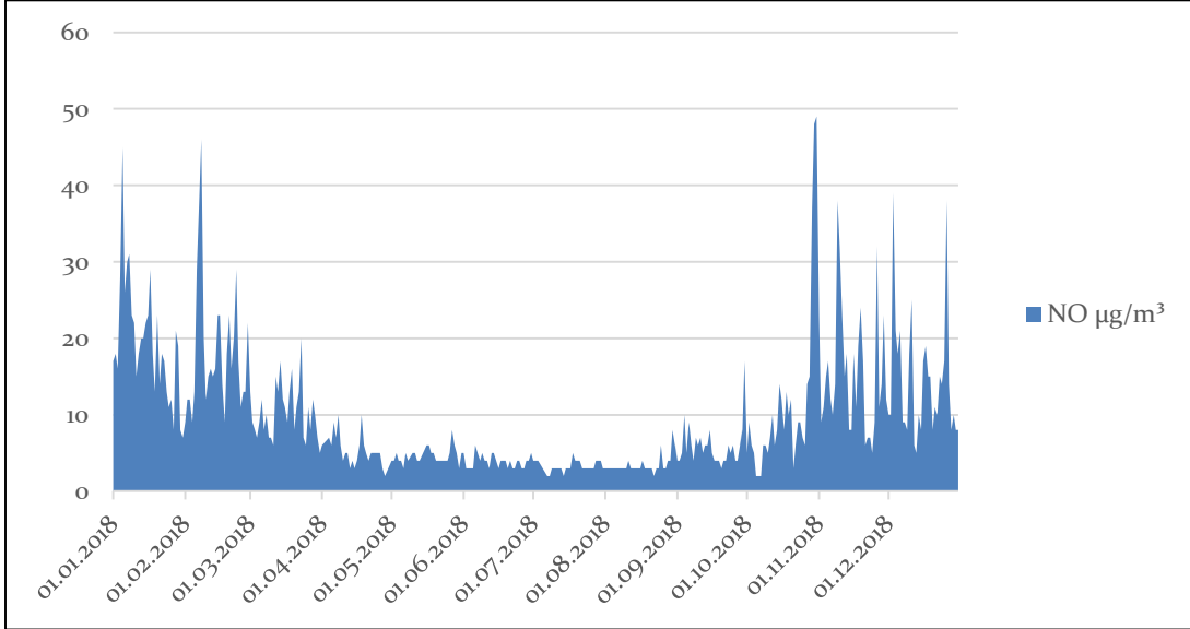
Grafik A.9 - Ağrı ili Doğubayazıt istasyonu NO parametresi günlük ortalama değer grafiği (havaizleme.gov.tr, 2019)
