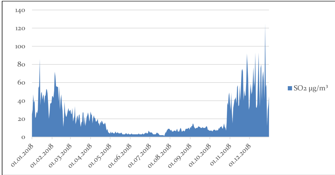
Grafik A.15 - Ağrı ili Patnos istasyonu SO 2 parametresi günlük ortalama değer grafiği (havaizleme.gov.tr, 2019)
