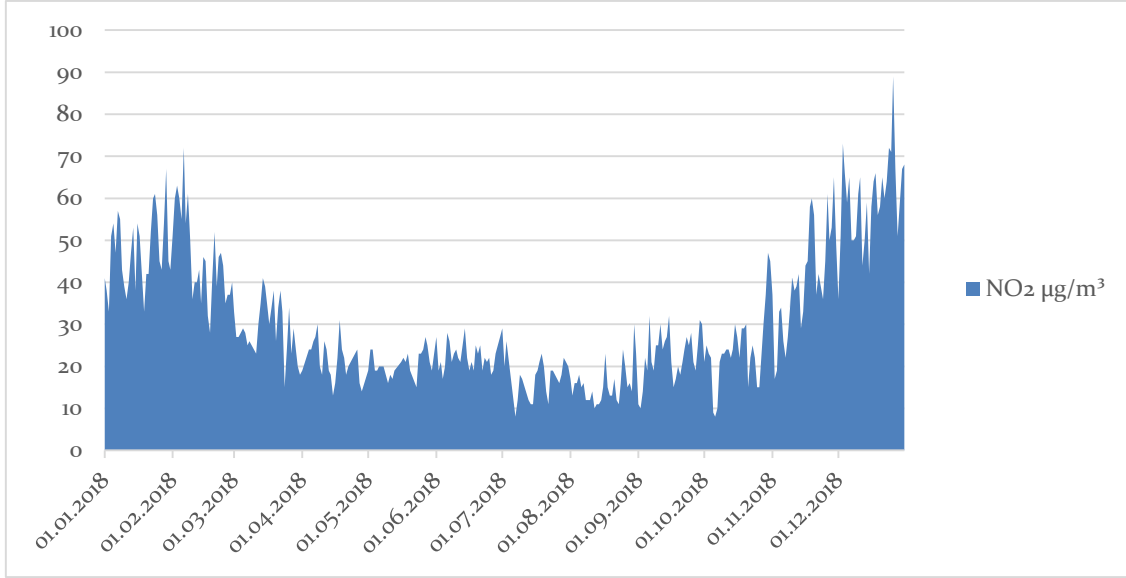
Grafik A.10 - Ağrı ili Doğubayazıt istasyonu NO 2 parametresi günlük ortalama değer grafiği (havaizleme.gov.tr, 2019)
