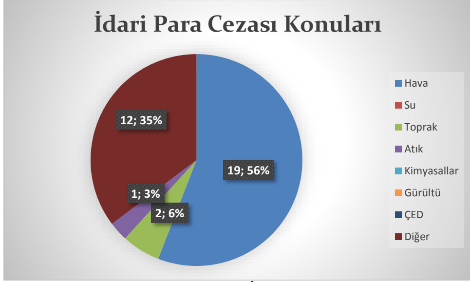
Grafik G.30 – Ağrı ilinde 2018 yılında ÇŞİM tarafından uygulanan idari para cezalarının konulara göre dağılımı (Ağrı ÇŞİM, 2019)
