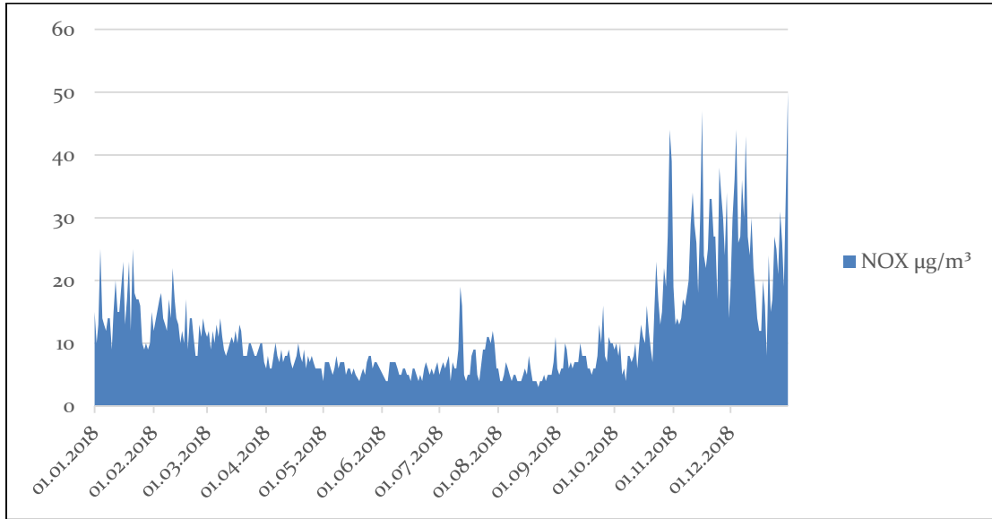
Grafik A.5 - Ağrı ili Merkez istasyonu NO x parametresi günlük ortalama değer grafiği (havaizleme.gov.tr, 2019)
