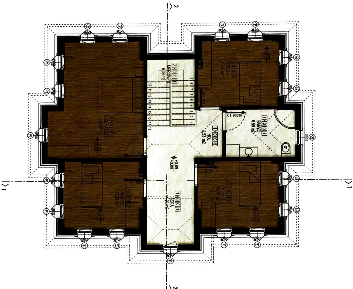
1. KAT PLANI BRÜT A:90.20 m 2 (balcon hariç) BRÜT A:90.20 m 2
