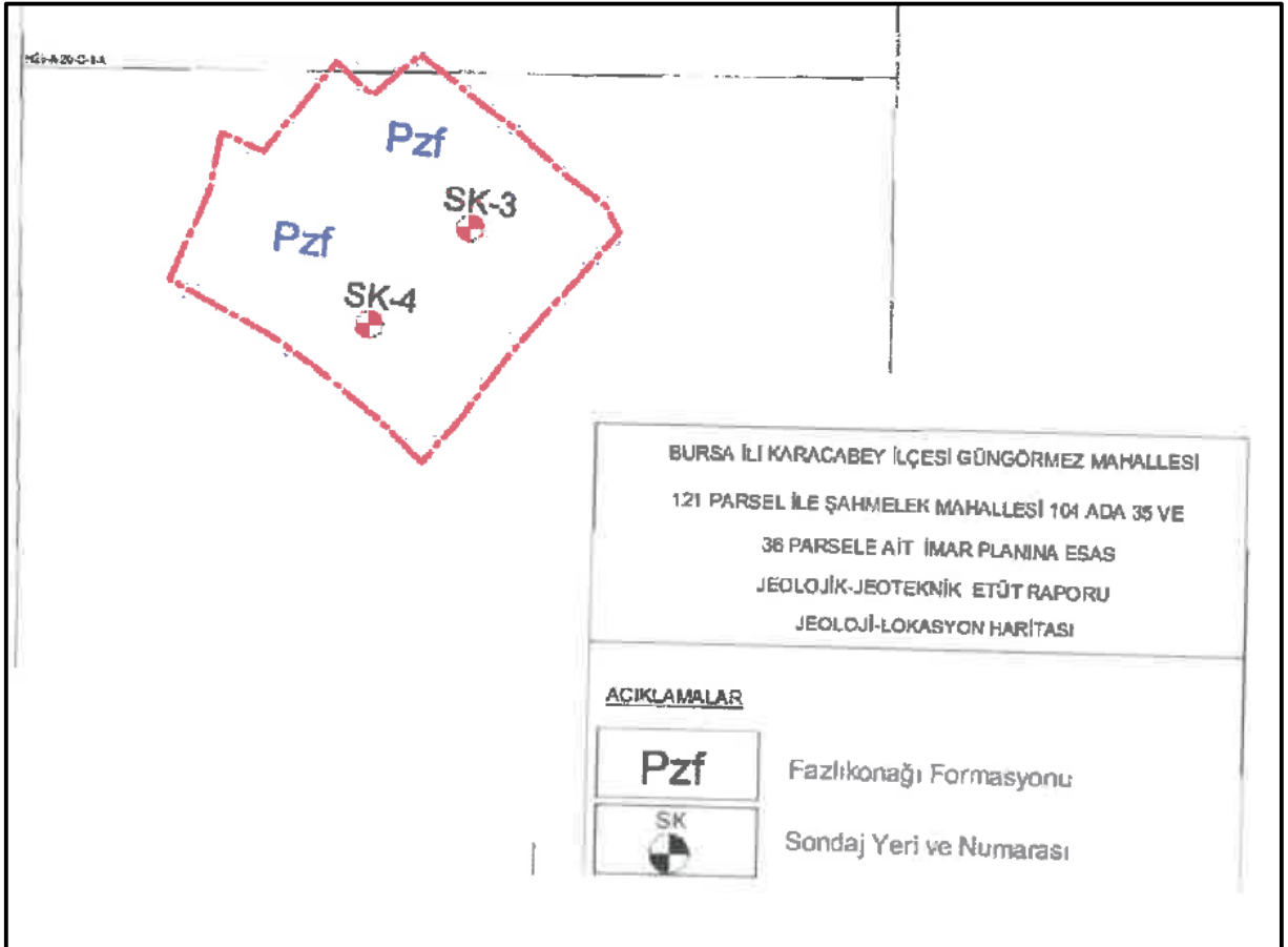
Şekil 8. Planlama Alanı Jeoloji Haritası
