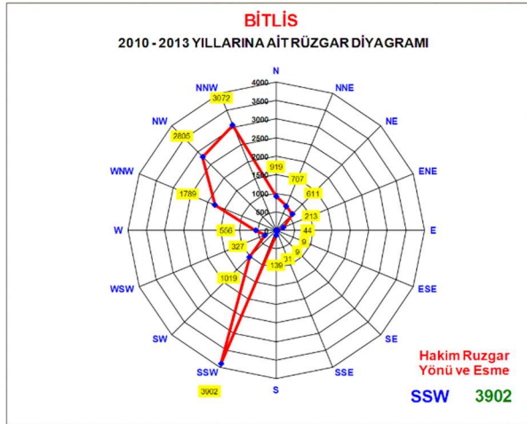
Şekil-3: Bitlis İline Ait Rüzgâr Diyagramı
