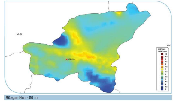
Şekil-4: Bitlis İli Rüzgâr Hızı Dağılımı
