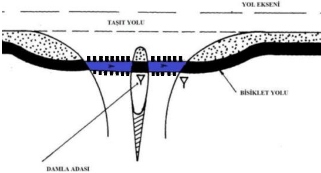
Şekil 4 - Damla adasından bisiklet yolu geçişi
