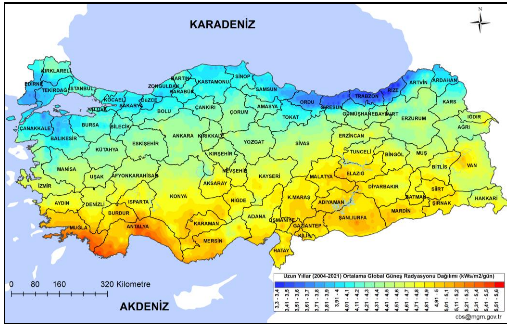
Şekil 1. Türkiye 2004-2021 Ortalama Global Güneş Radyasyonu (Enerjisi) Dağılımı (kW/m²/gün)
