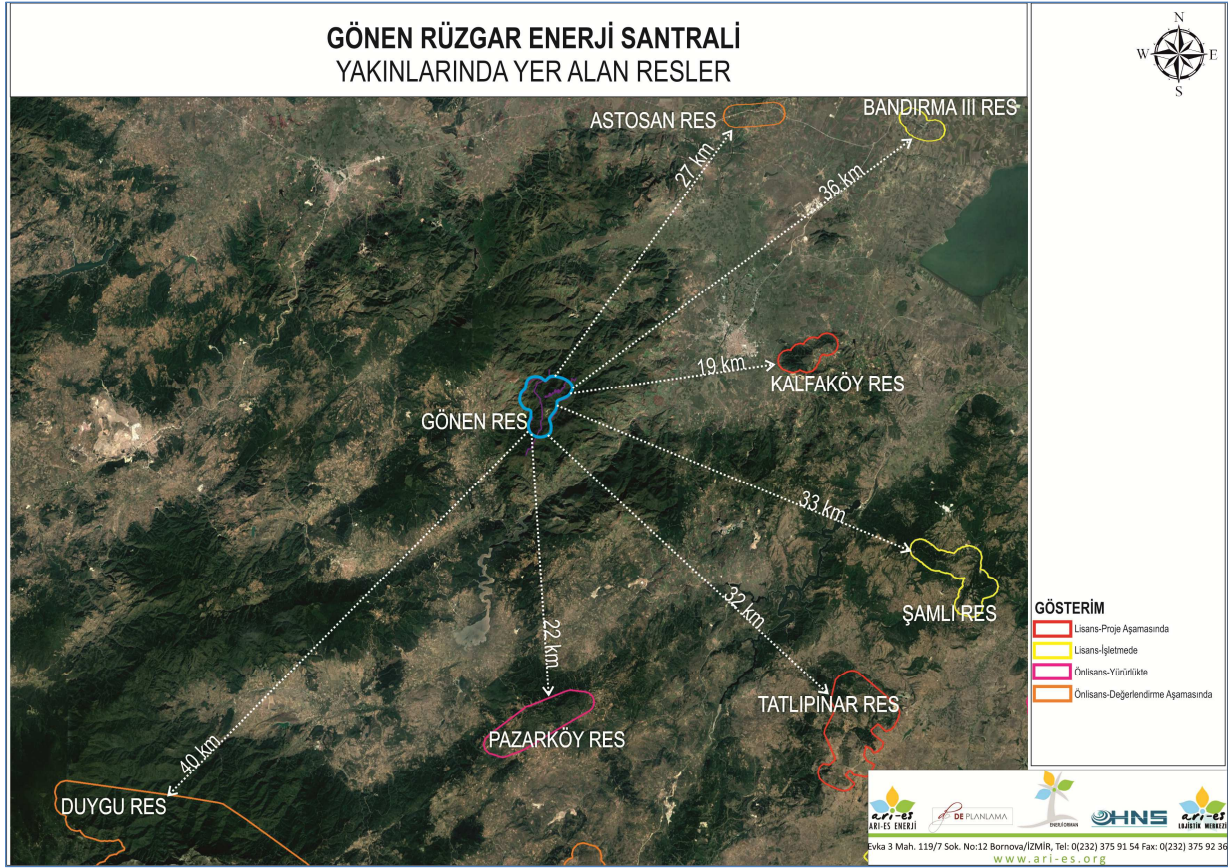
Şekil 18: Proje Sahası Çevresinde Yer Alan Rüzgar Santralleri
