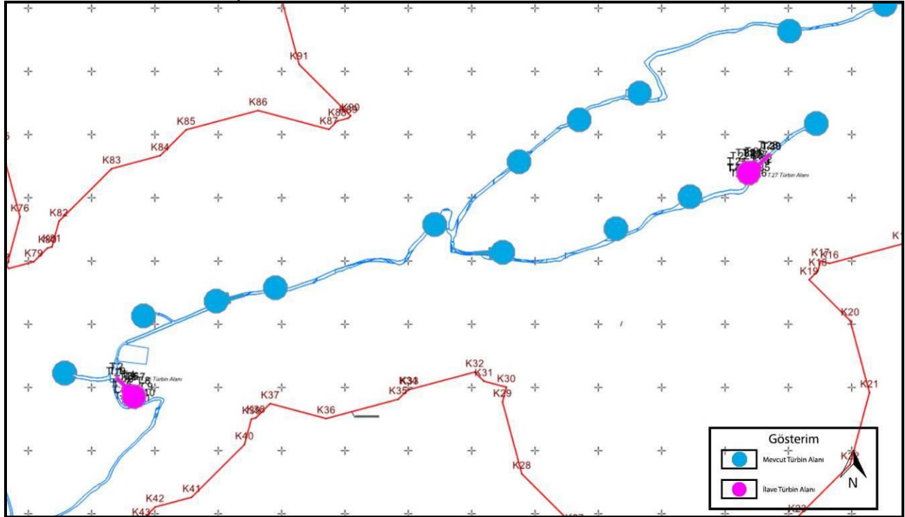
Şekil 5 - Orman Ön İzni Vaziyet Planı
