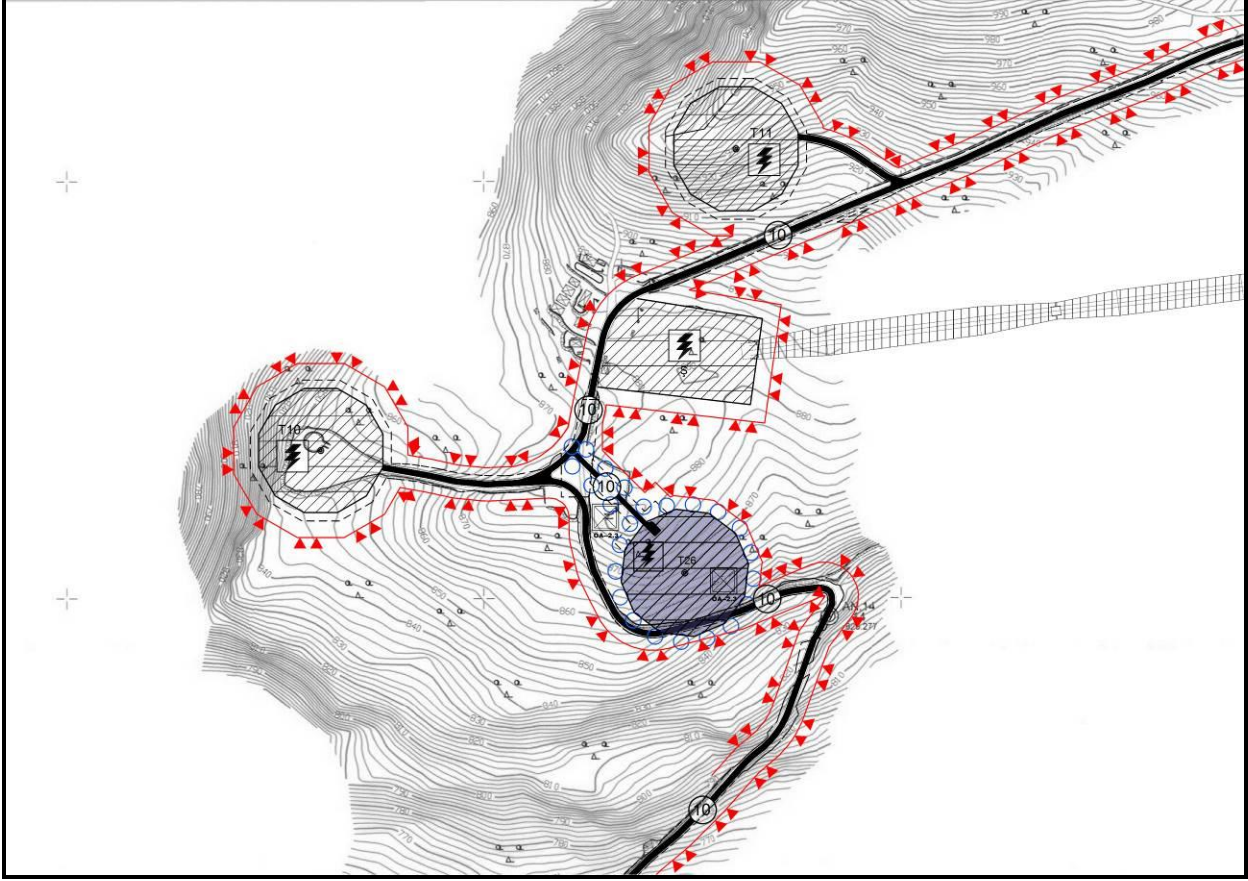
Şekil 11 - 1/5.000 Ölçekli İlave Nazım İmar Planı Önerisi
