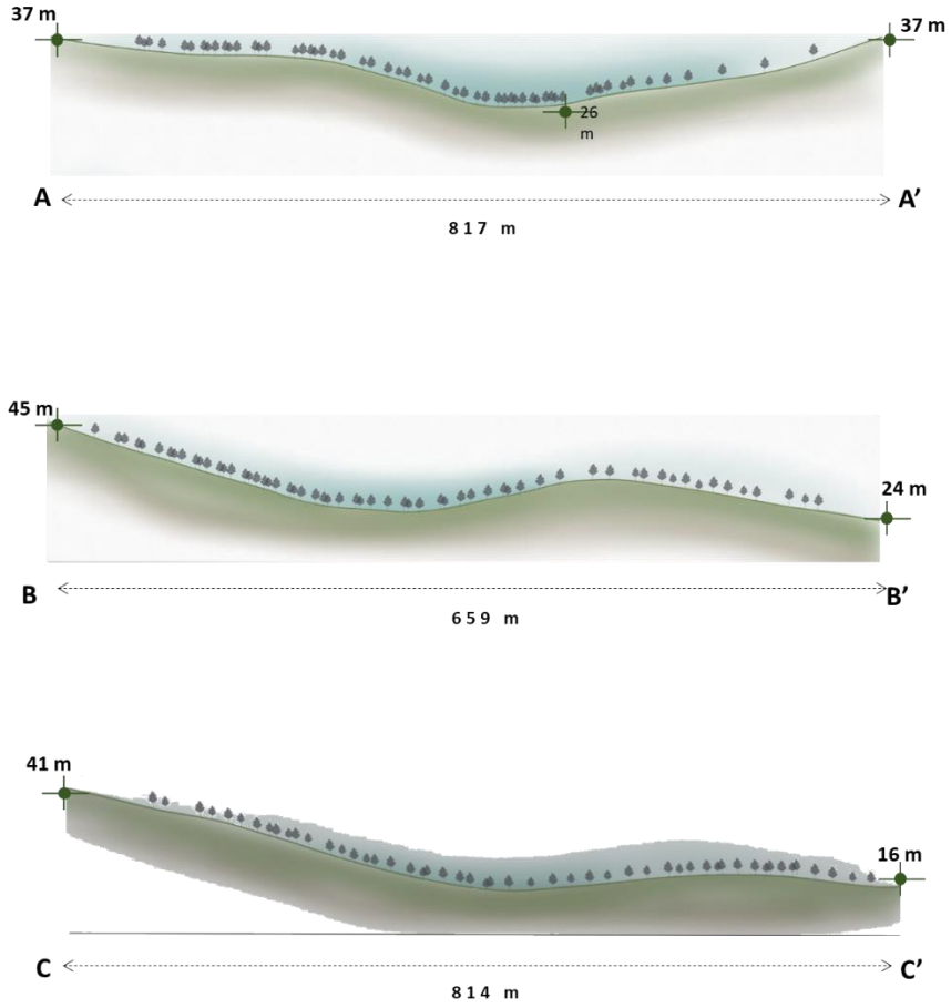
Şekil 22: Kesit Şeması
