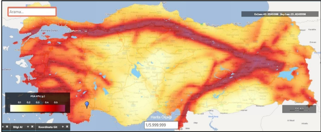
Şekil 9. Türkiye deprem tehlike haritası
