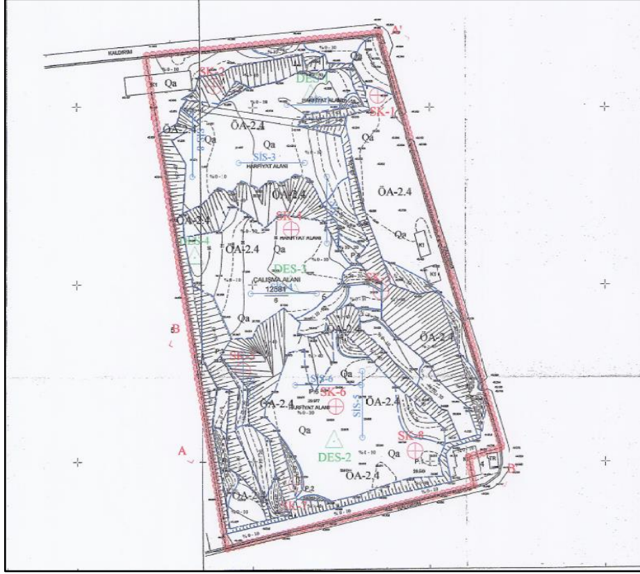
Şekil 3. İmar Planına Esas Jeolojik – Jeoteknik Etüt - Yerleşime Uygunluk Haritası
