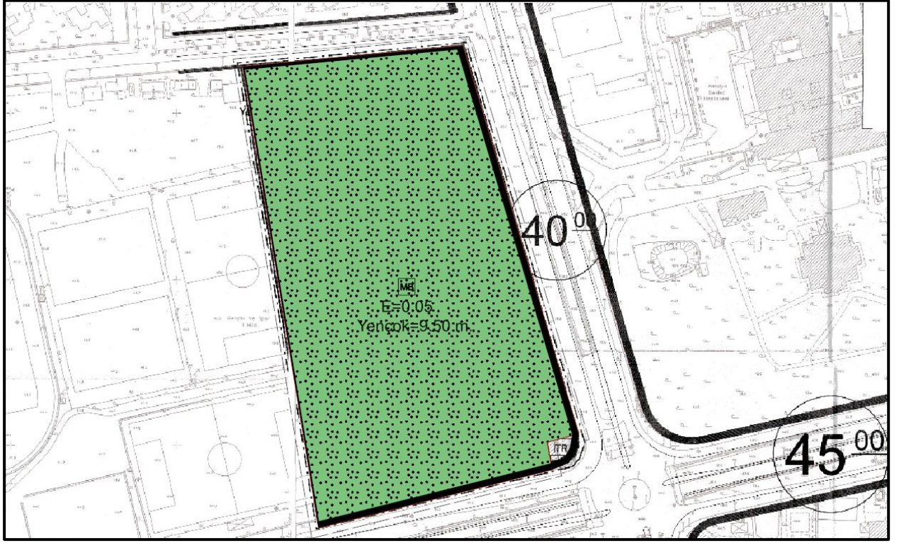
Şekil 7: Planlama Alanına İlişkin 1/1000 Ölçekli Uygulama İmar Planı Teklifi
