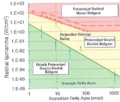
Şekil 1. Parlama Tehlikesi Grafiği: Retinal ışıltama ve kaynaktan gelen ışık demetinin geliş açısının bir fonksiyonu olarak parlama etkisini gösterir grafik [1].
