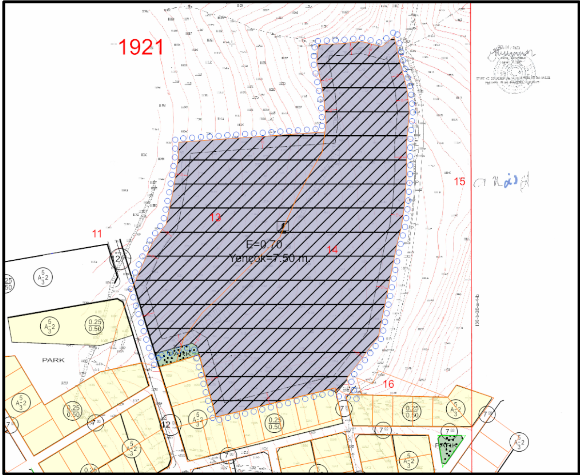
Şekil 7. 1/1000 Ölçekli Uygulama İmar Planı
