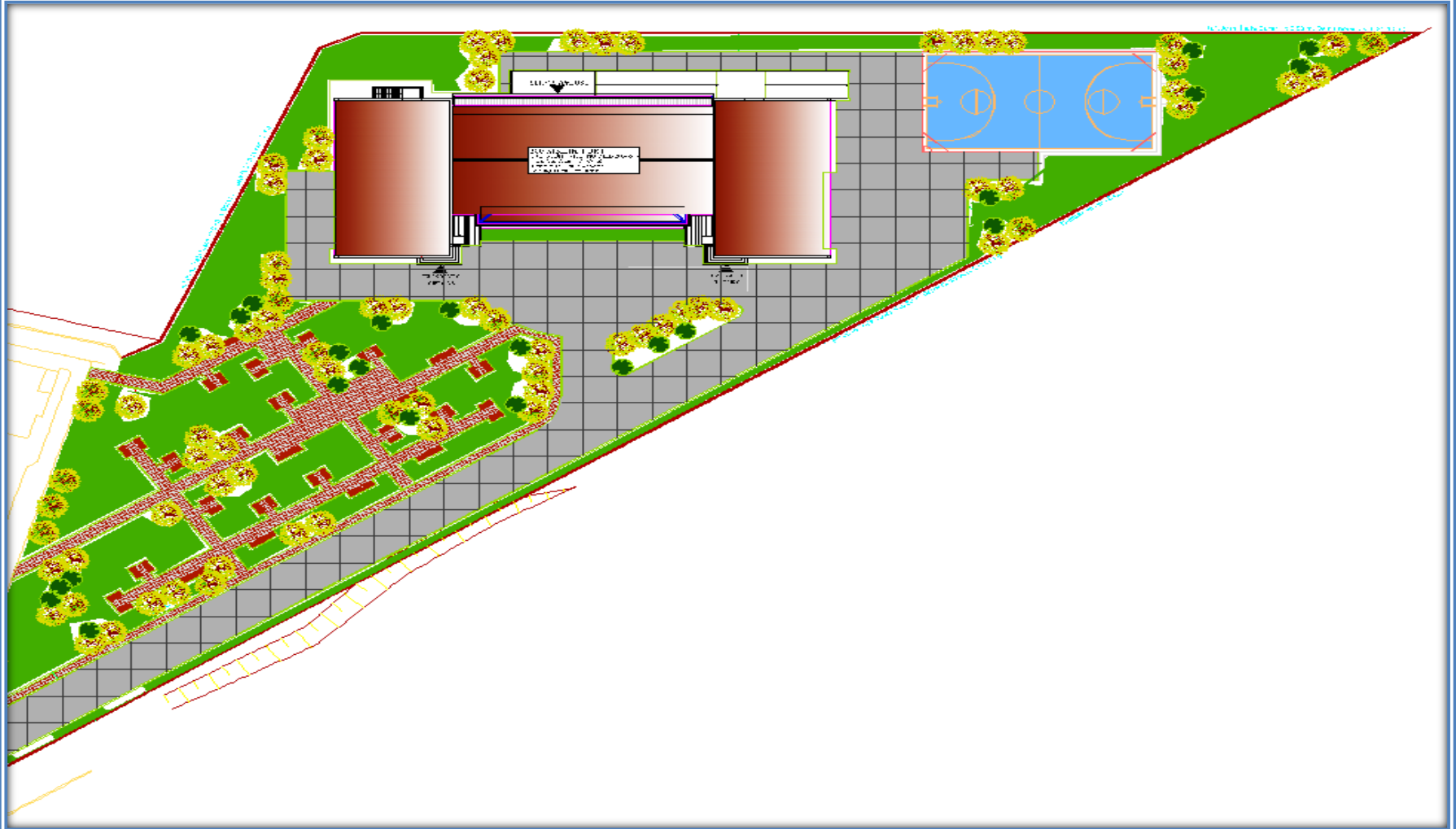
VAZİYET PLANI
