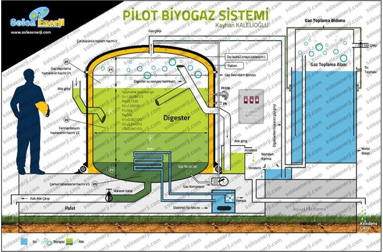
Şekil 5 - Biyogaz üretimi şeması
