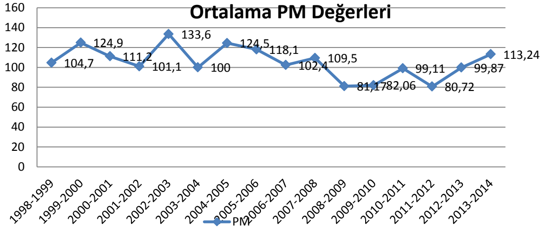
Grafik 1.3-2 Uzun yıllar hava ölçüm sonuçları ortalaması (PM)
