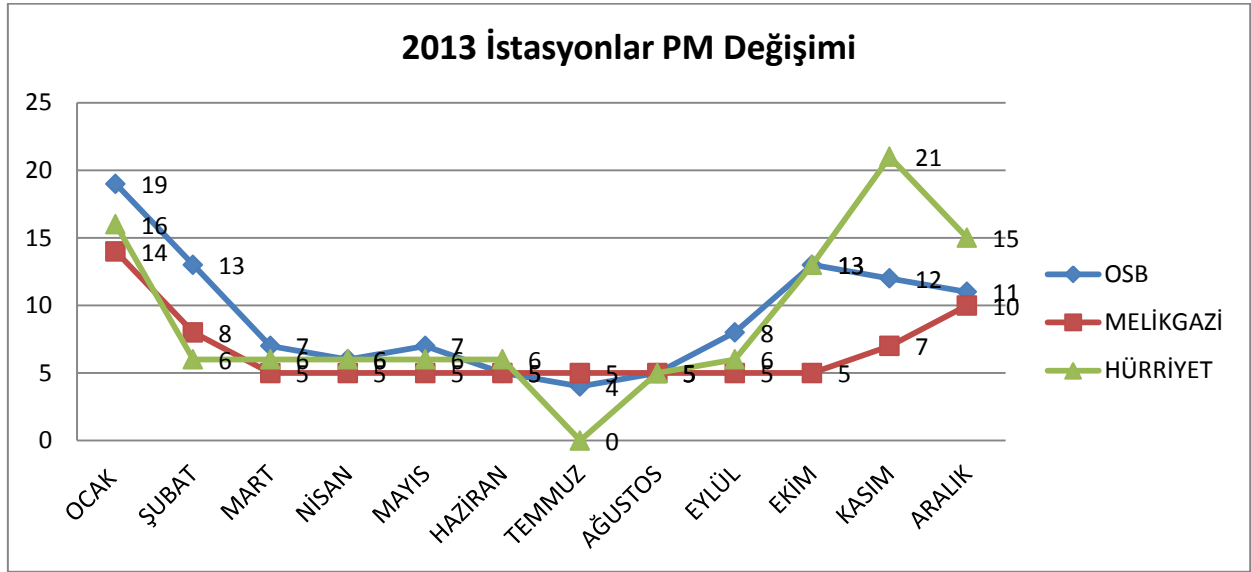
Grafik A.4- İlimizde 3 İstasyonu Parametresi Günlük Ortalama Değer Grafiği PM(Ölçülen Tüm Parametreler İçin Ayrı Grafik Konulacaktır)
