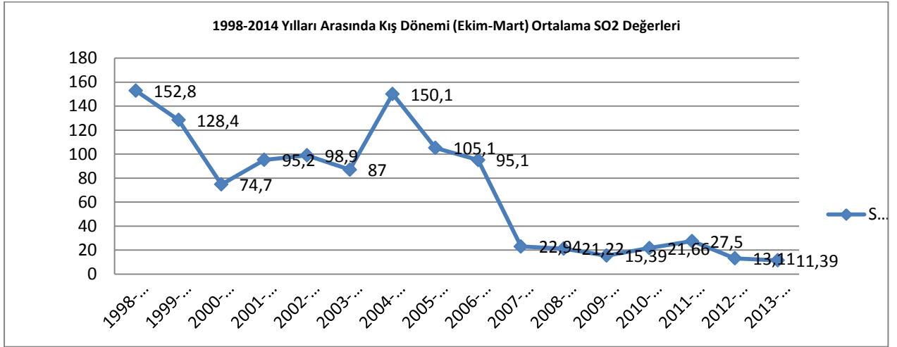
Grafik A-2 Kayseri 1998-2013 yılları arası SO 2 Değerleri Değişimi
