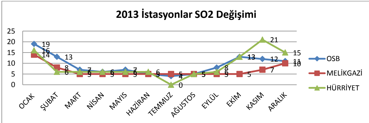
Grafik A.3- İlimizde 3 İstasyonu Parametresi Günlük Ortalama Değer Grafiği SO 2 (Ölçülen Tüm Parametreler İçin Ayrı Grafik Konulacaktır)
