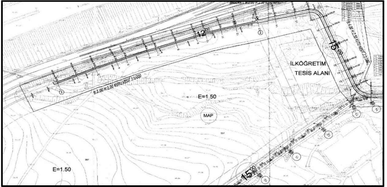
Şekil 14: 2012 tarih ve 23024 sayılı onaylı Dere Islahı Uygulama Projesi
