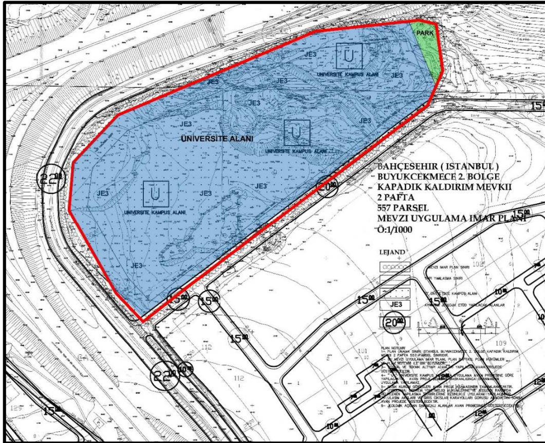
Şekil 9: 27.10.2003 t.t. 1/1000 ölçekli Mevzi Uygulama İmar Planı
