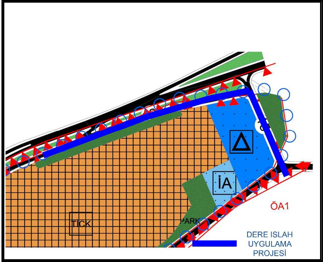
Şekil 16: 1/5000 Ölçekli Nazım İmar Planı ve Dere Islah Uygulama Projesi
