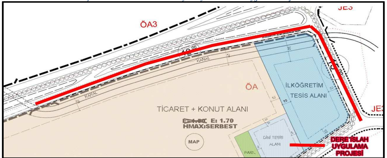
Şekil 15: 01.04.2013 t.t. İmar Planında Yer Alan Dere Güzergahı ve Dere Islah Uygulama Projesi
