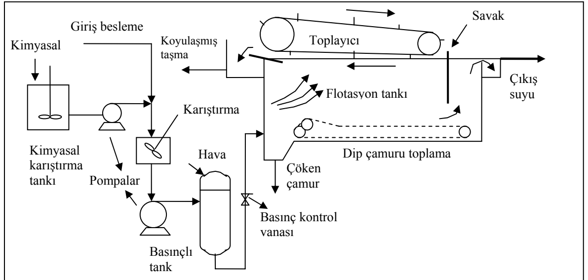
Şekil 4.9. Çözülmüş hava ile yüzdürme sistemi (DAF) şematik görünümü
