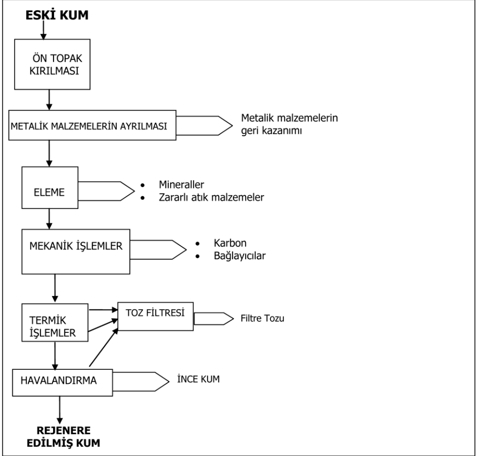
Şekil 5.2 Termik eski kum geri kazanım tesisi
