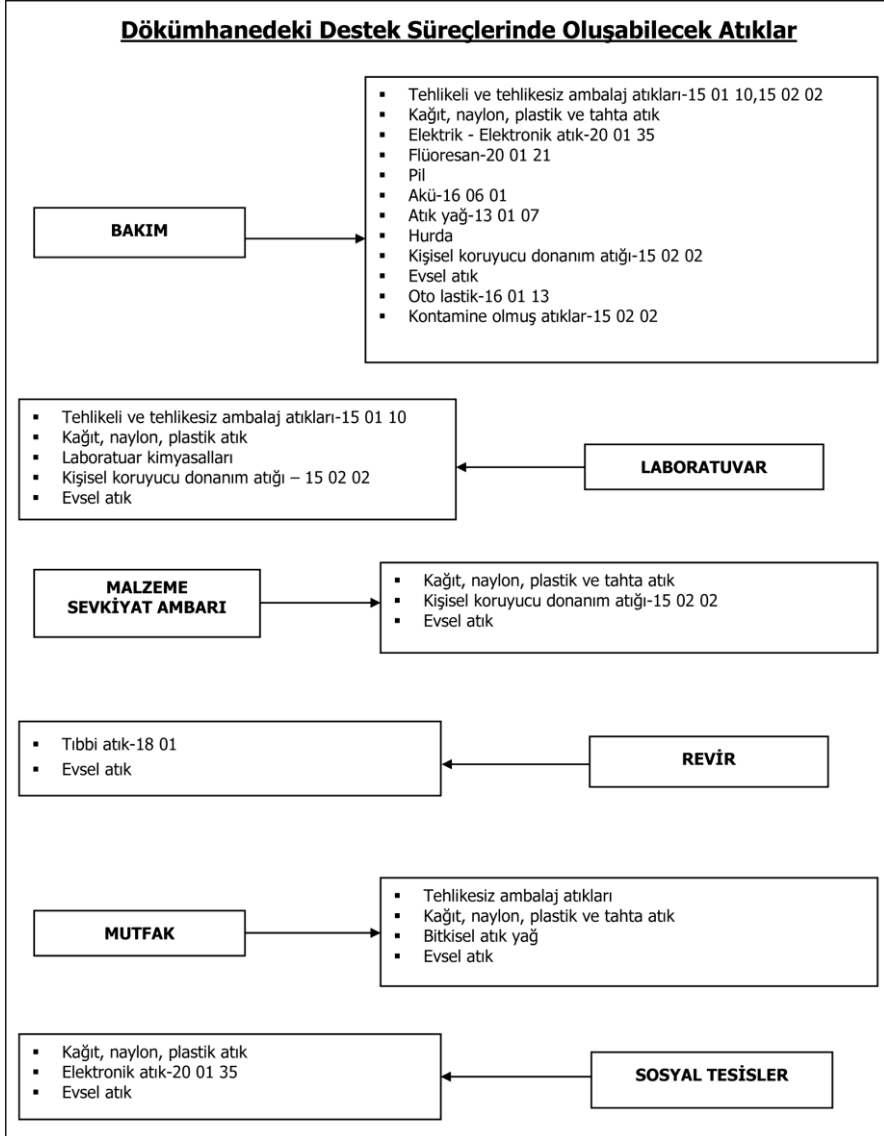
Şekil 4.3 Dökümhanelerde yan işlemlerde oluşabilecek atıklar
