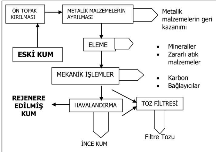
Şekil 5.1 Mekanik eski kum geri kazanım tesisi
