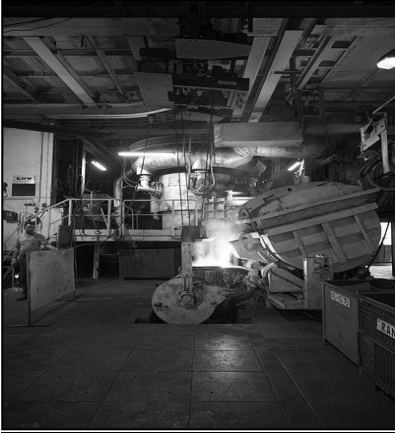
Resim 3.1 Kupol ocağında ergitme
