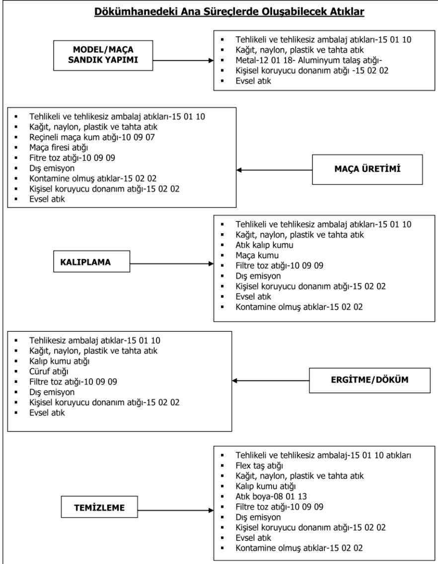
Şekil 4.2 Dökümhanelerde temel işlemlerde oluşabilecek atıklar
