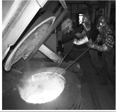
Resim 3.2 Elektrikli ocakta ergitme
