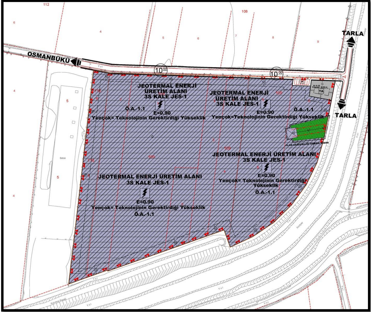
Şekil 1: 1/1000 Ölçekli Uygulama İmar Planı
